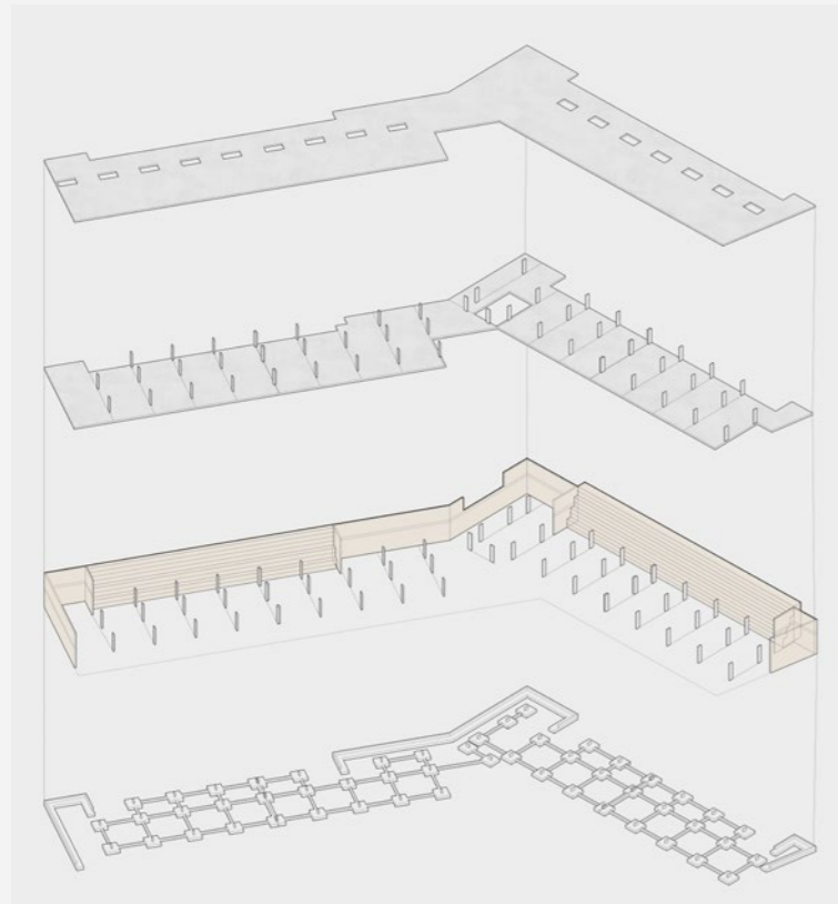
Muros de piedra en seco en el Pou Boronat
