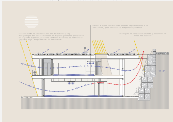
Comportamiento del edificio en verano
