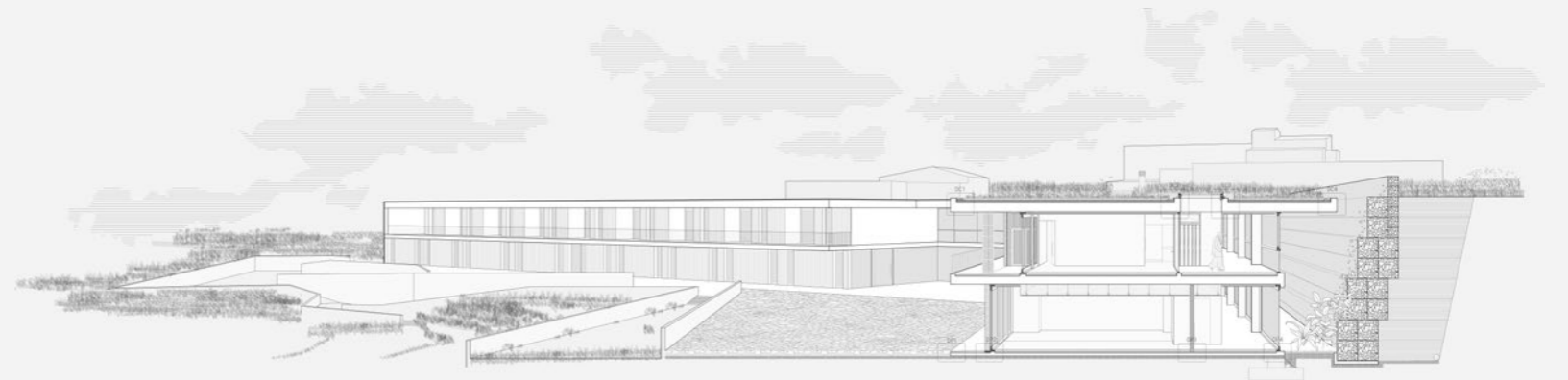
El conjunto | Sección fugada
