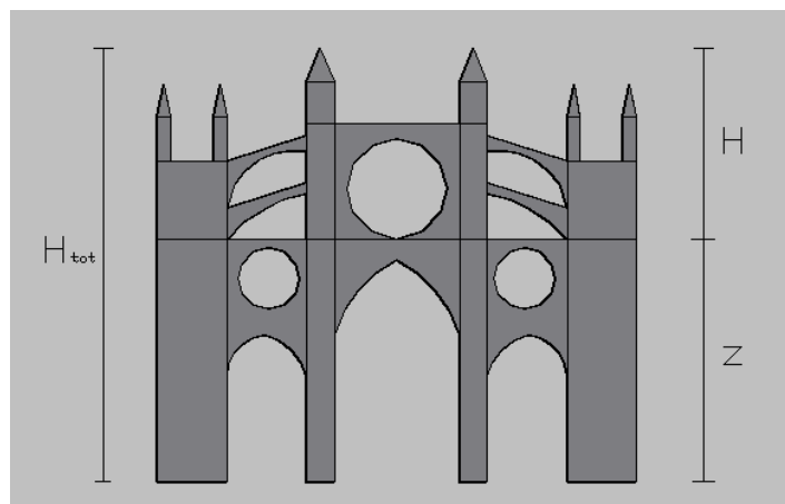
Figure A2 – Geometrical parameters
