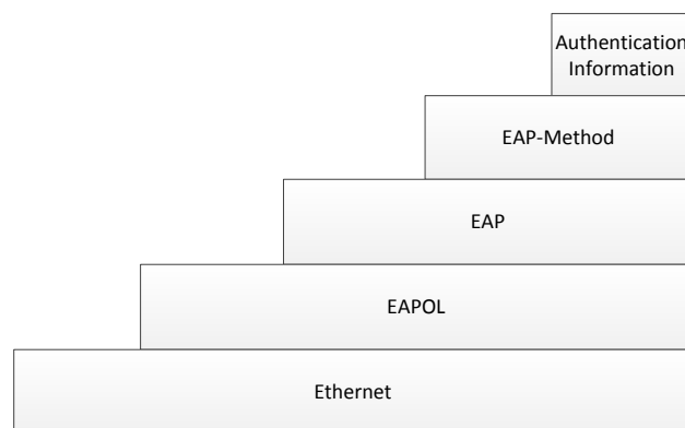
Figura 2.3 – Pila d'encapsulaments 802.1x
