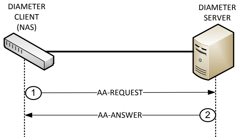
Figura 2.28 – La fase d'autenticació/autorització en Diameter
