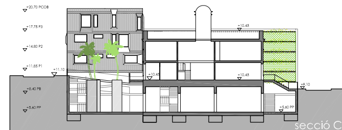
secció C
