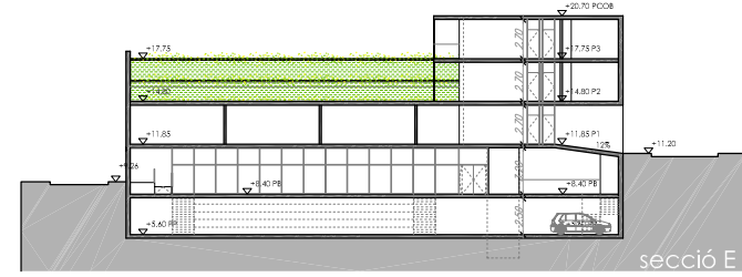
secció E
