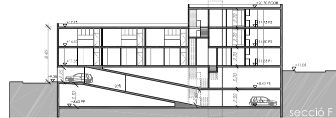
secció F
