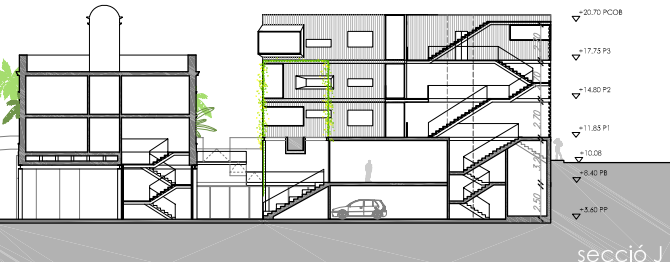
secció J
