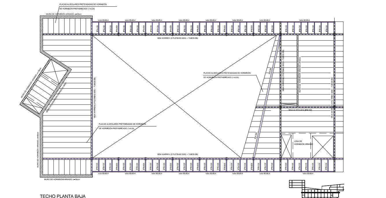
TECHO PLANTA BAJA
