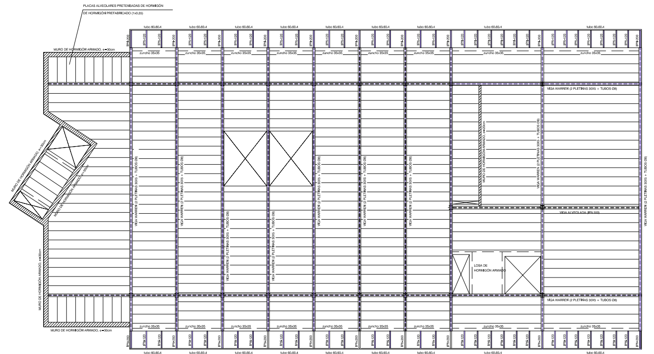
TECHO PLANTA PRIMERA
