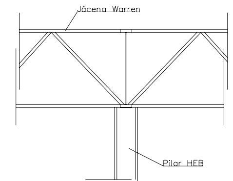
DETALLE UNION ENTRE VIGAS Y PILAR
