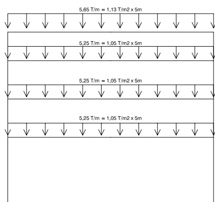
CARGAS PÓRTICO
