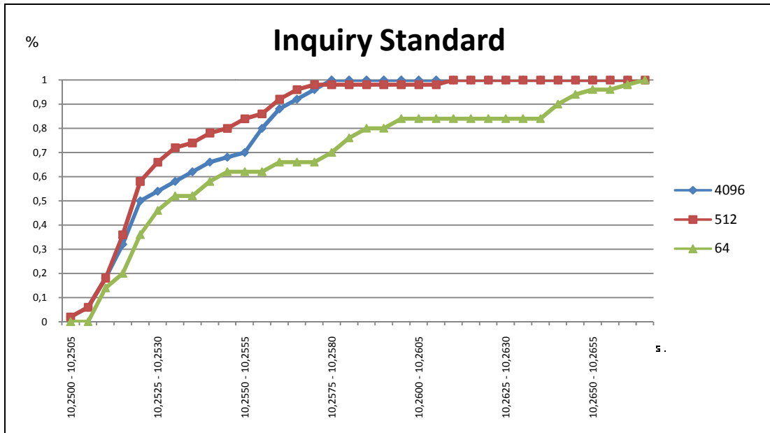
Fig. 3.2.5. Tiempo de conexión Inquiry Standard
