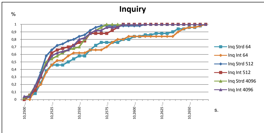
Fig. C.1. Tiempo de conexión Inquiry
