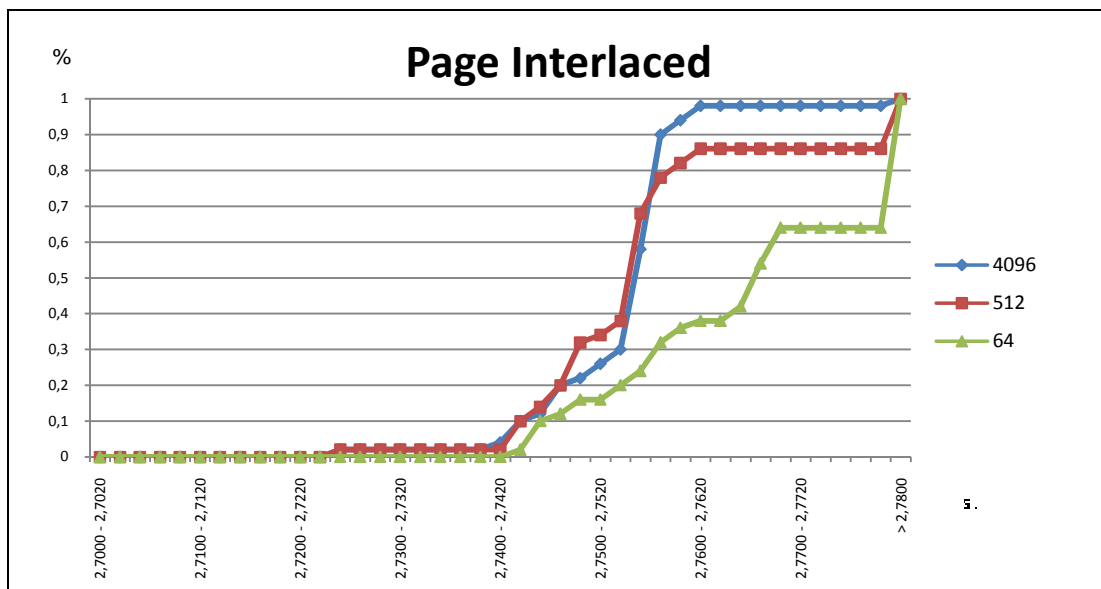
Fig. 3.2.8. Tiempo de conexión Page Interlaced
