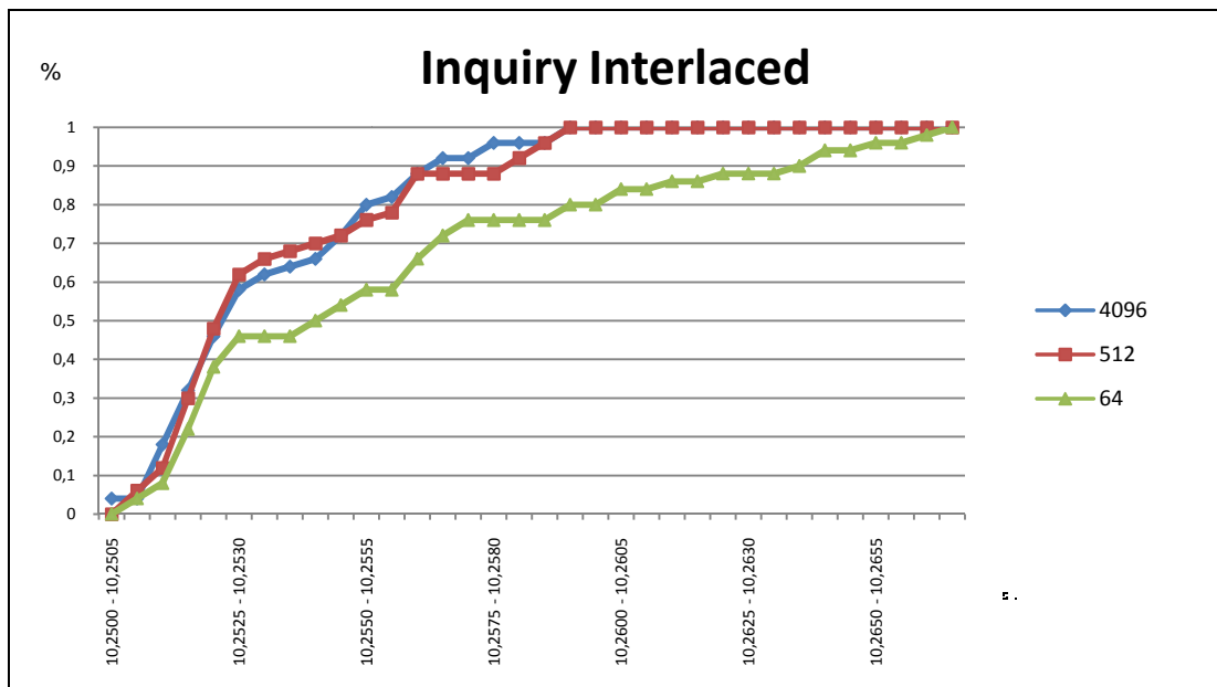
Fig. 3.2.6. Tiempo de conexión Inquiry Interlaced
