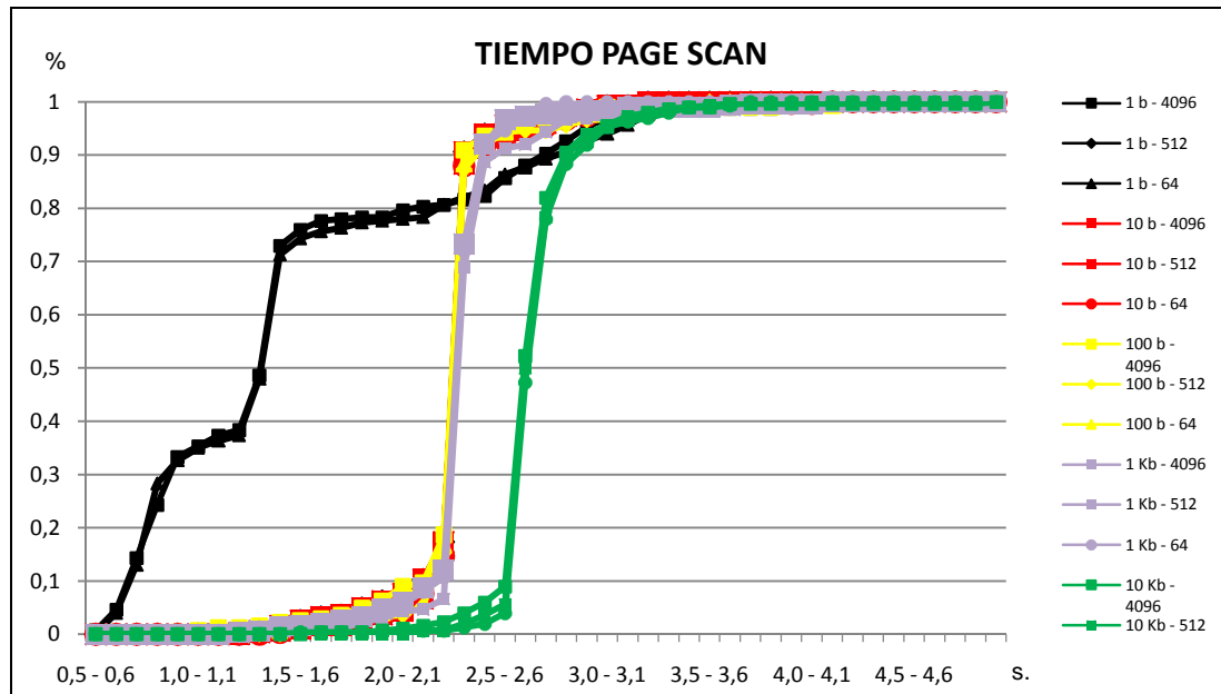
Fig. 3.2.10. Gráfica acumulativa modo page
