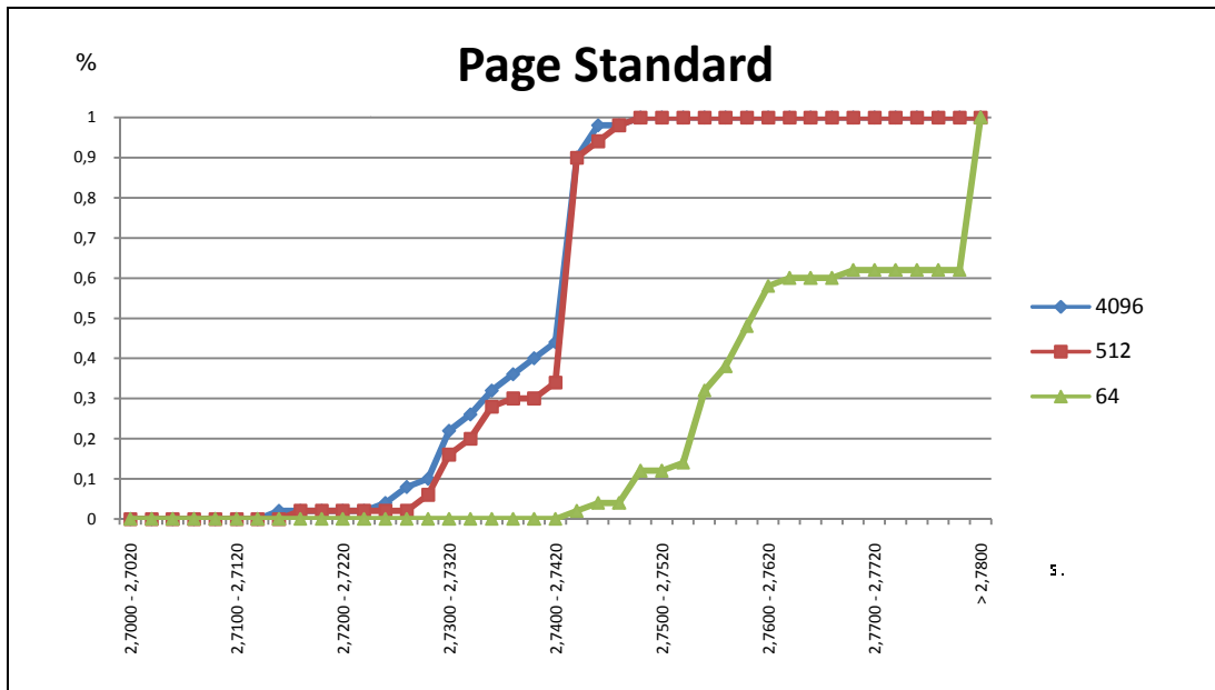
Fig. 3.2.7. Tiempo de conexión Page Standard
