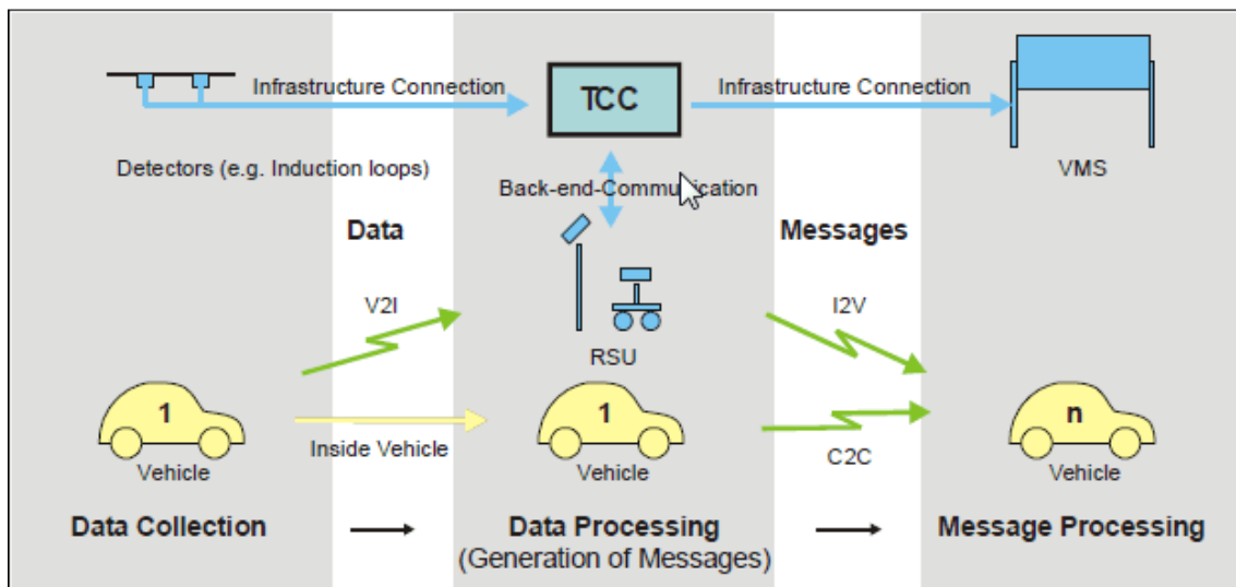
Fig. 1.1.1 Esquema de un sistema V2R
