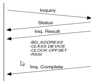
Fig. 3.2.3. Proceso de inquiry
