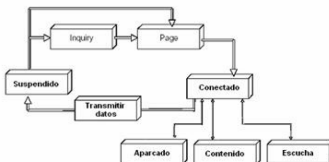
Fig. 3.2.4. Establecimiento de conexiones Bluetooth
