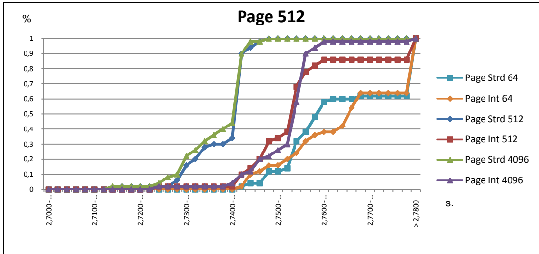
Fig. C.2. Tiempo de conexión Page
