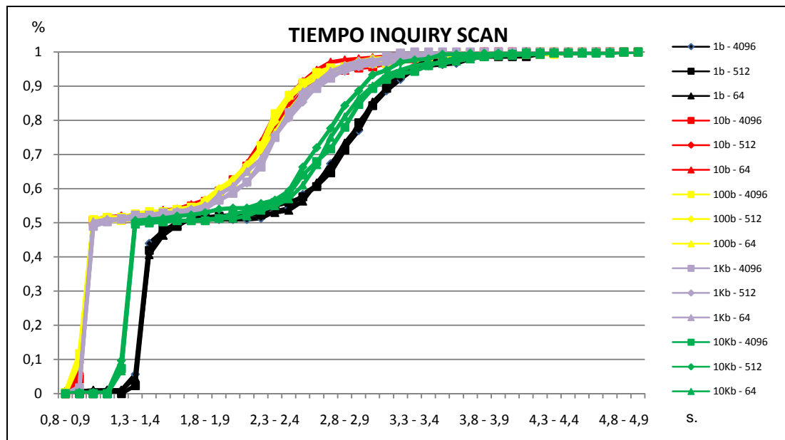
Fig. 3.2.9. Gráfica acumulativa modo inquiry
