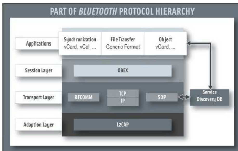
Fig. 3.2.2. Pila de protocolos Bluetooth
