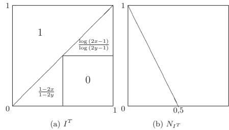
Figura 2: Estructura de la implicación I^T y su negación natural N_{I^T} cuando T = ((0, 1/2, T_L), (1/2, 1, T_P)) .
