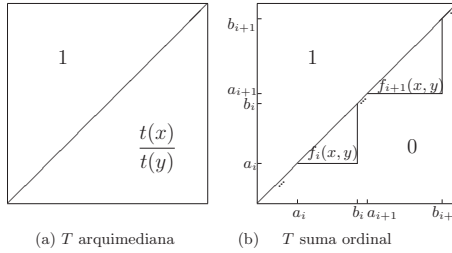
Figura 1: Estructura de las implicaciones I^T cuando T es arquimediana y cuando es la suma ordinal T = ((a_i, b_i, T_i))_{i \in I} . Se denota por f_i(x, y) = \frac{t_i\left(\frac{x-a_i}{b_i-a_i}\right)}{t_i\left(\frac{y-a_i}{b_i-a_i}\right)} para todo i \in I .
