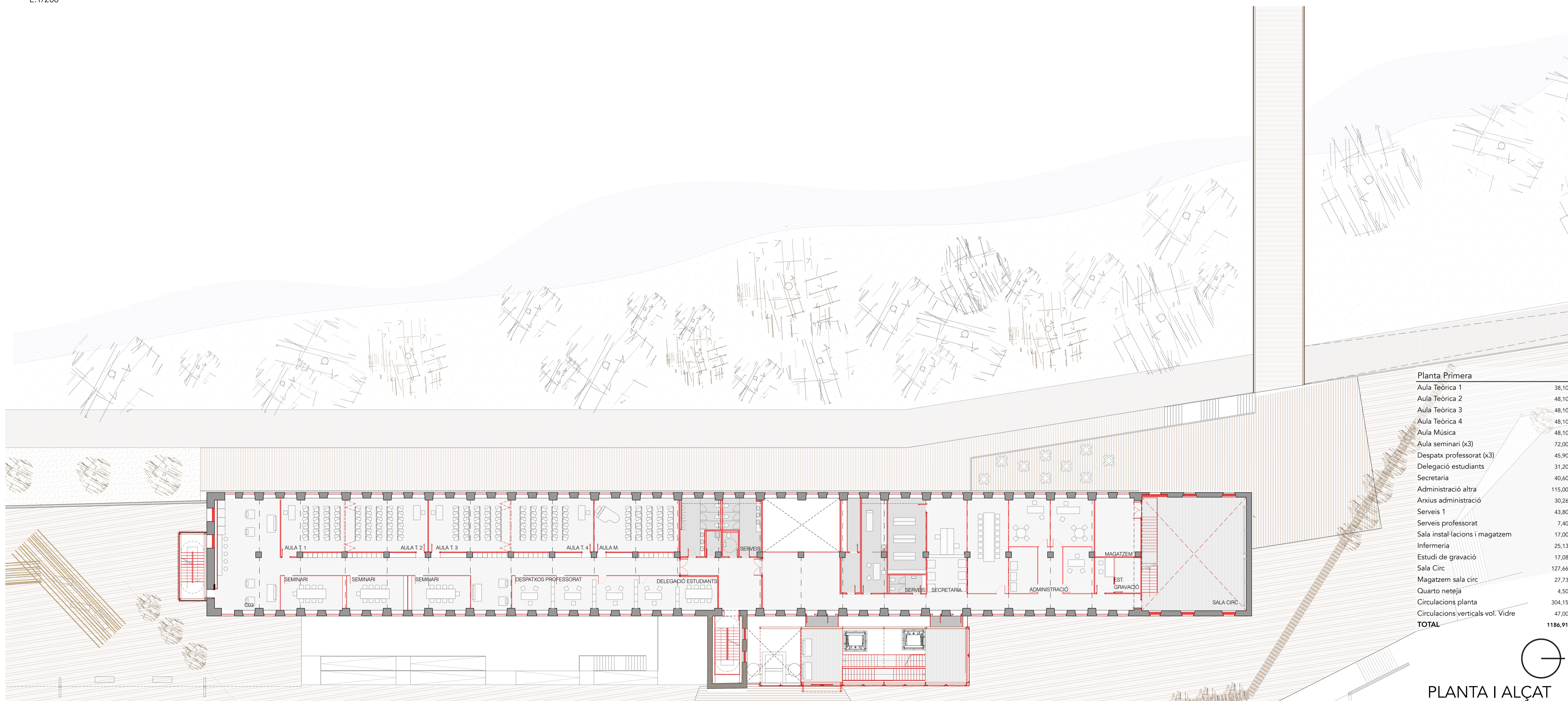
PLANTA PRIMERA(+214,42) E:1/200
