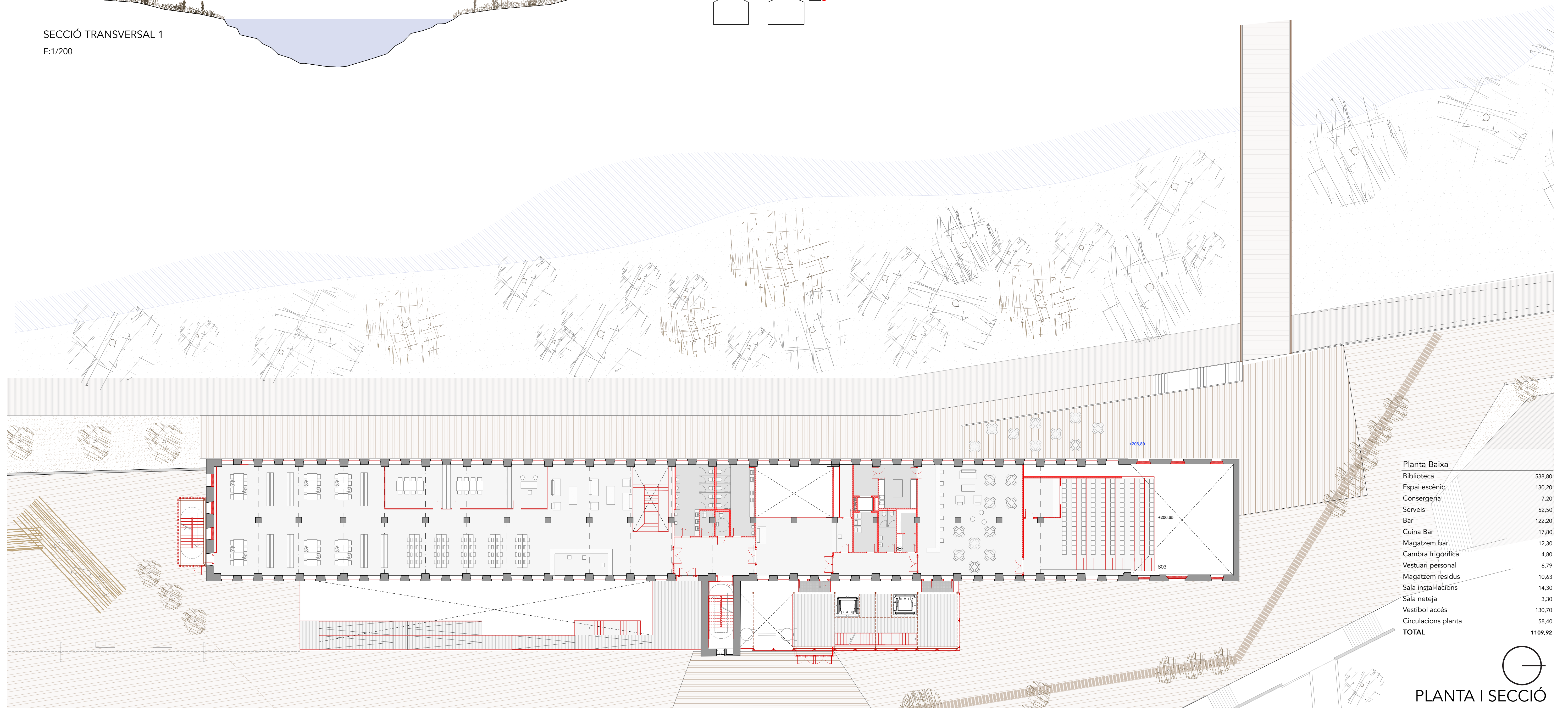
PLANTA BAIXA (+210,35) E:1/200
