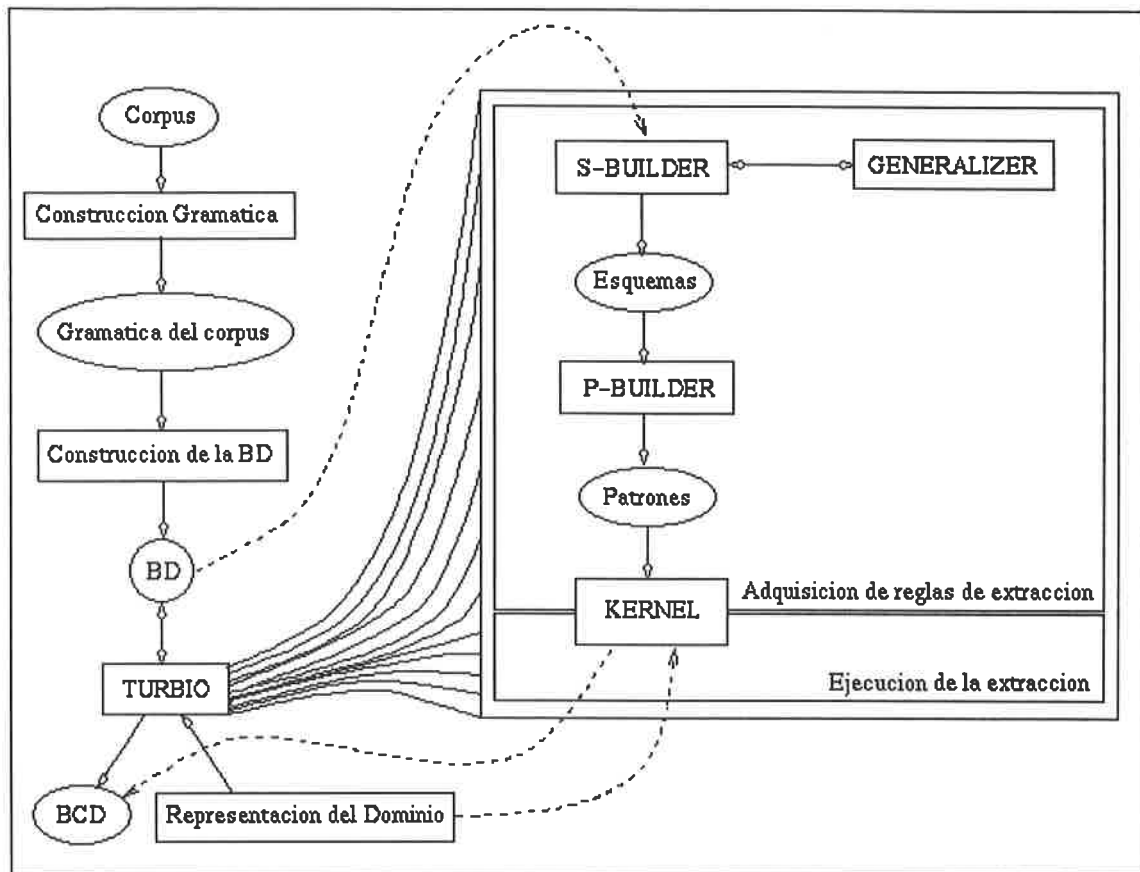
Fig. 2.- Entorno y arquitectura de TURBIO
