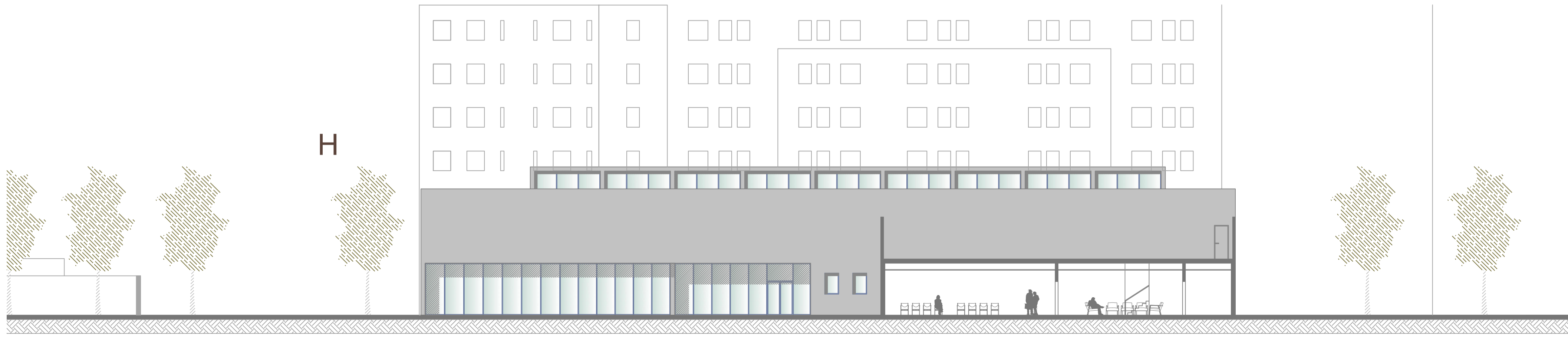
ARQUITECTURA: 9 SECCIONES LONGITUDINALES E 1:200
