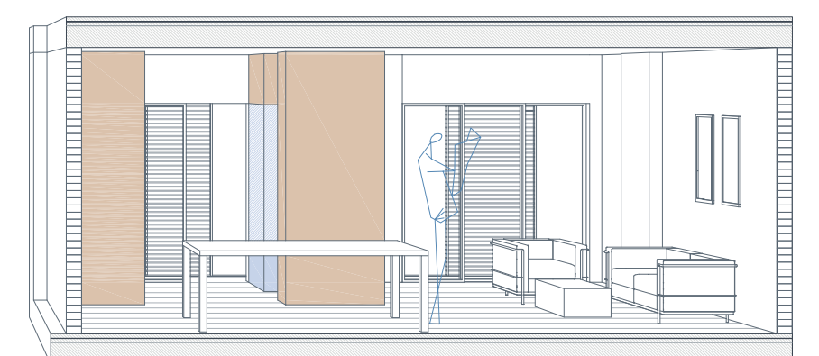
ALZADOS INTERIORES E_1:50
