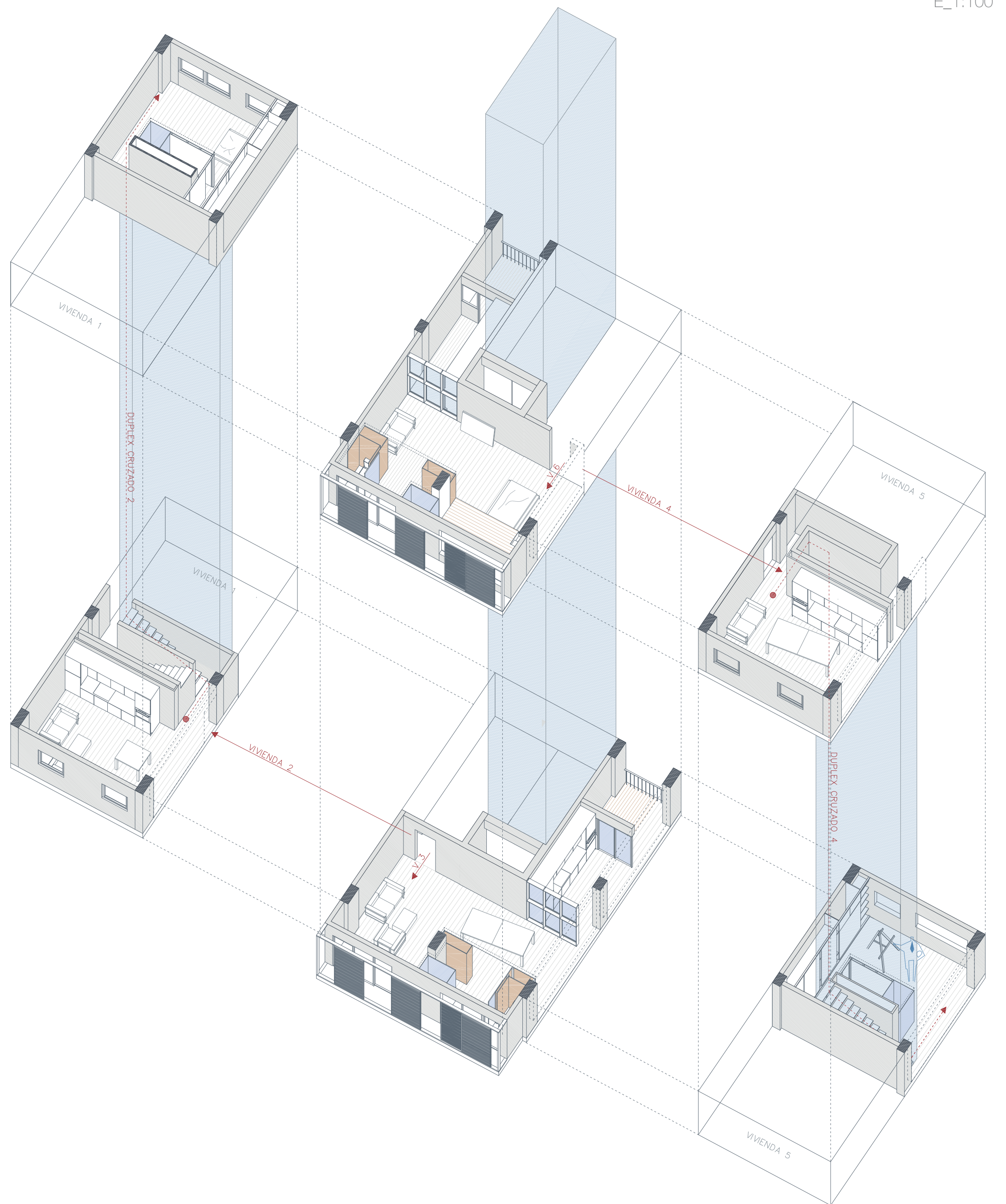
AXONOMETRÍA EXPLOTADA E_1:100
