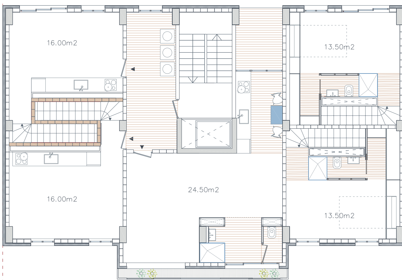
PLANTA TIPO 2 E_1:100
