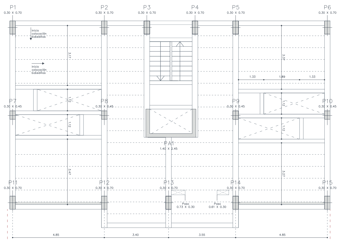
PLANTA INTERVENCIÓN ESTRUCTURAL E_1:100
