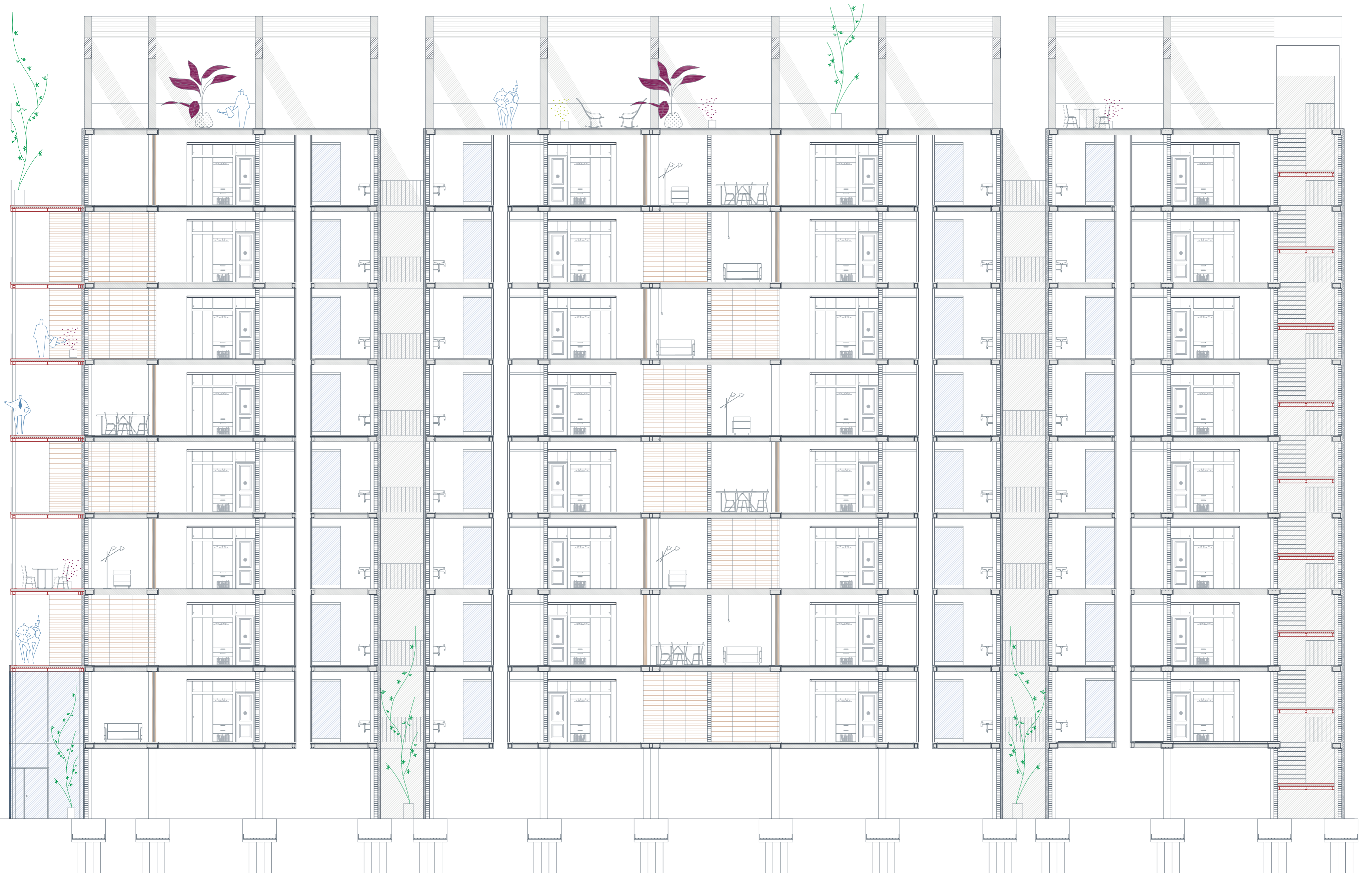
SECCIÓN LONGITUDINAL B E_1:100
