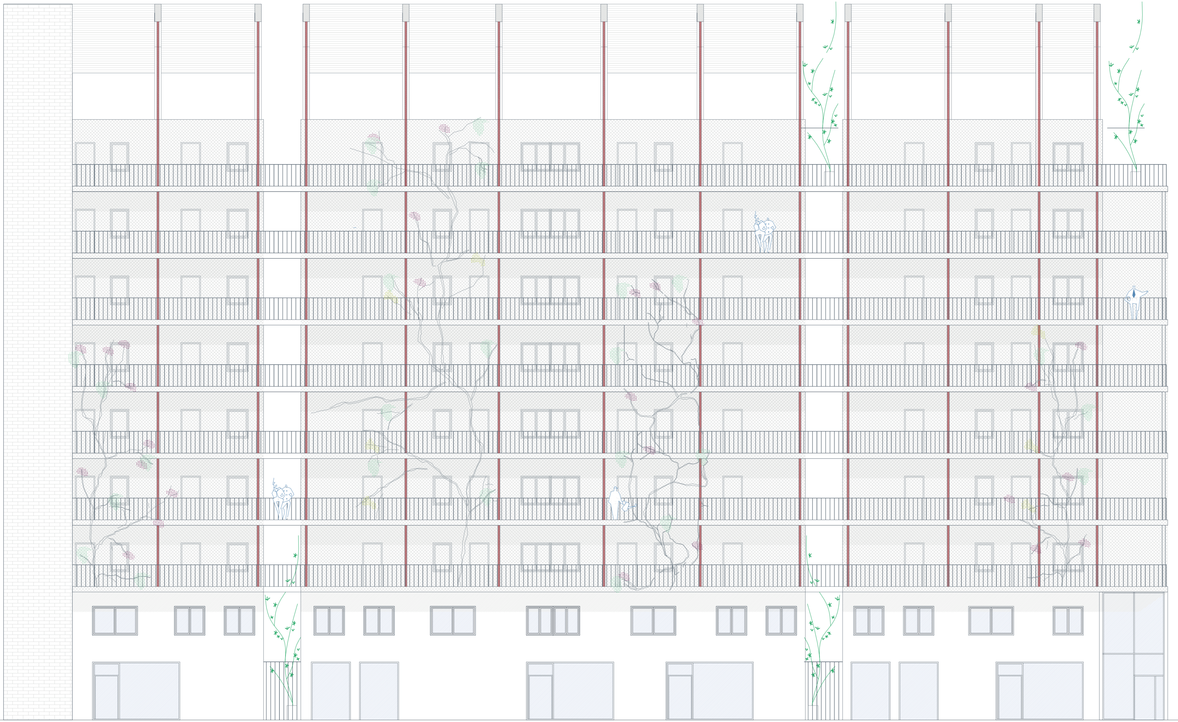
ALZADO PASARELA E_1:100
