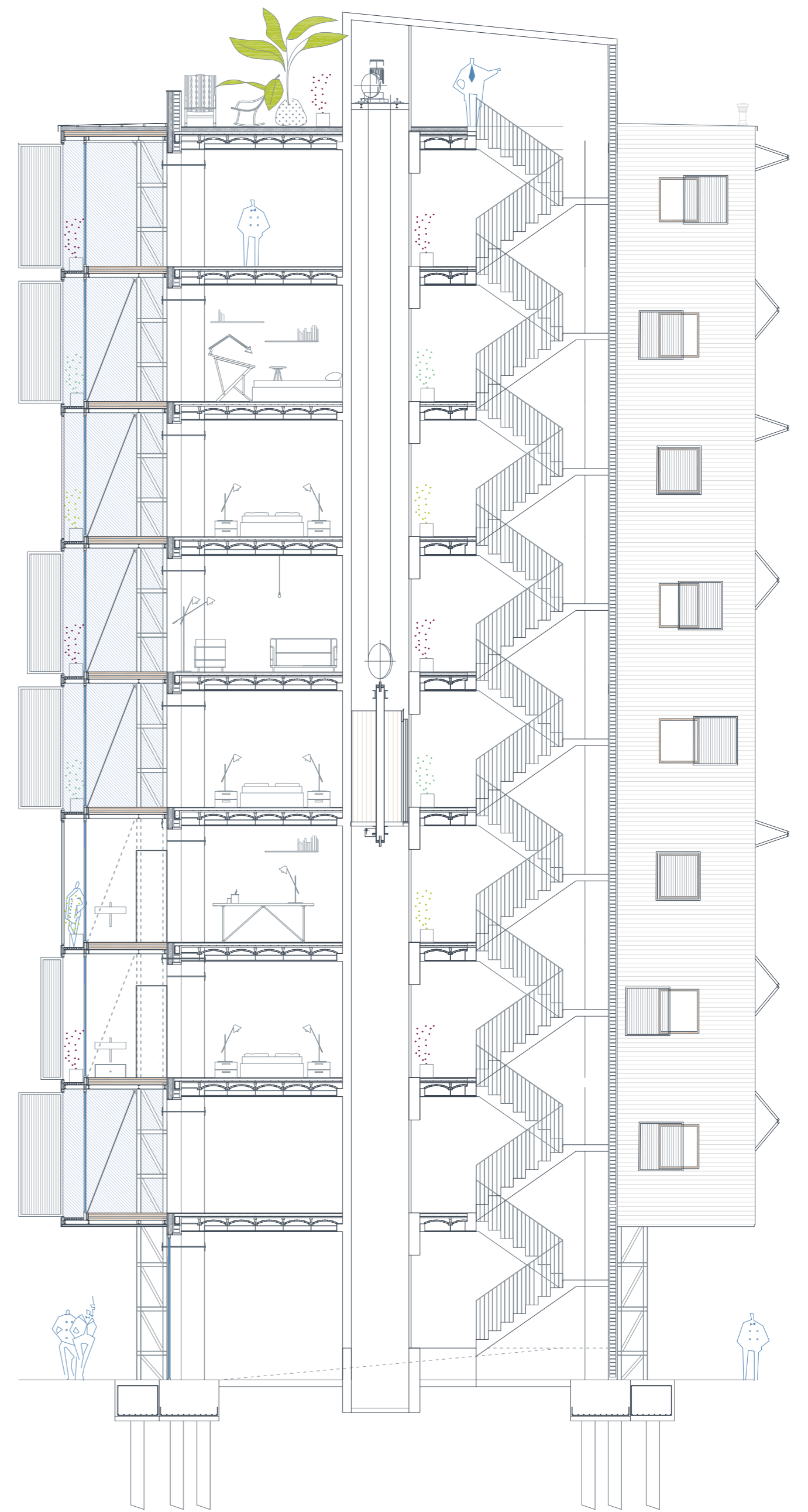
SECCIÓN TRANSVERSAL A E_1:100
