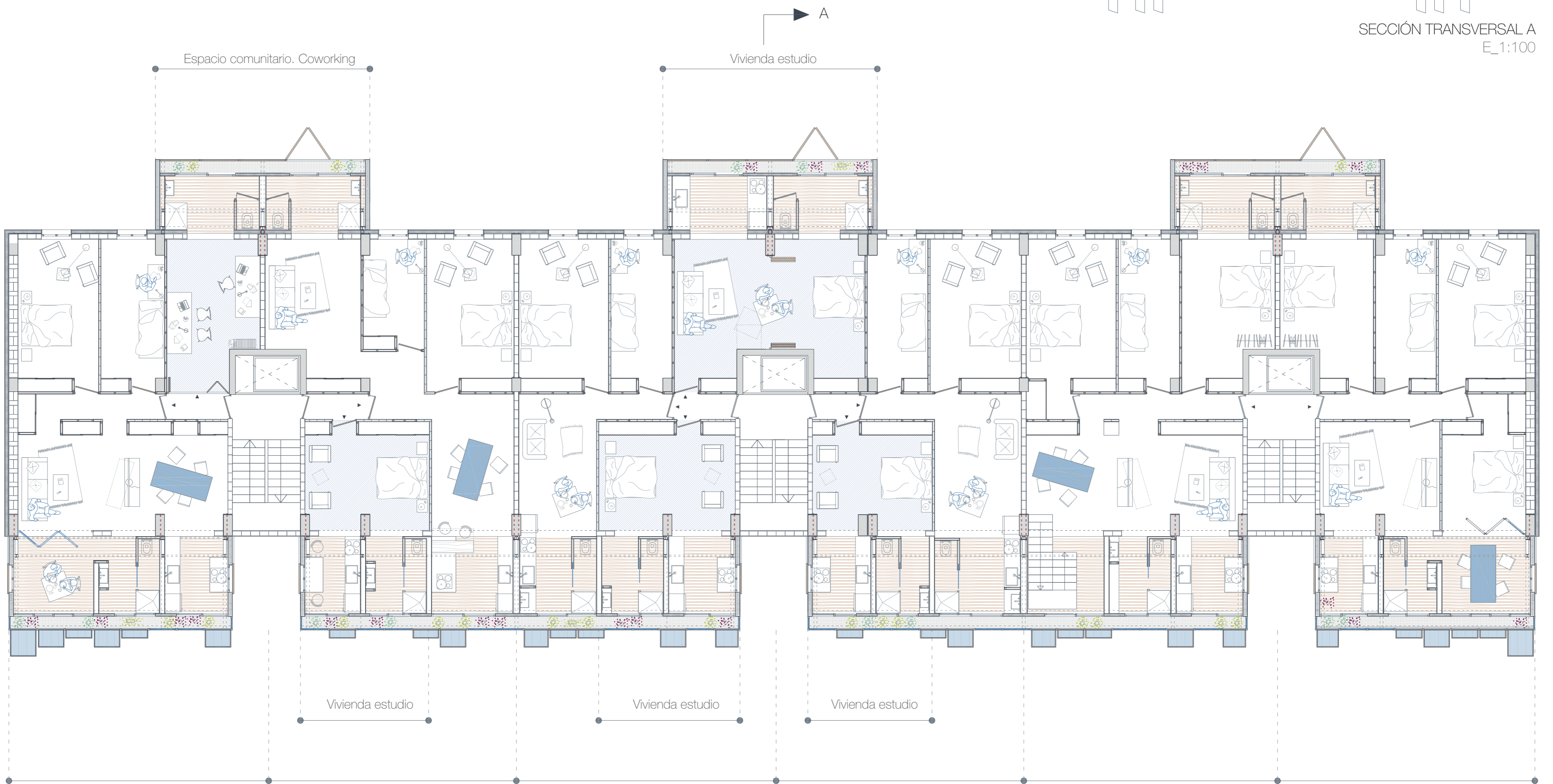
PLANTA 1. APLICACIÓN DEL SISTEMA E_1:100
