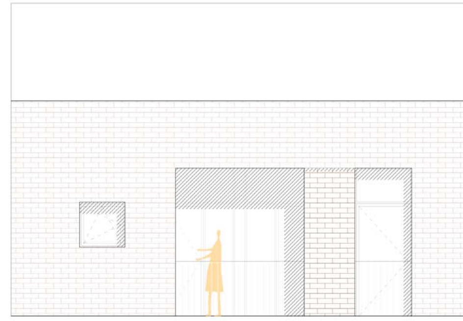
ALÇAT A-A'
