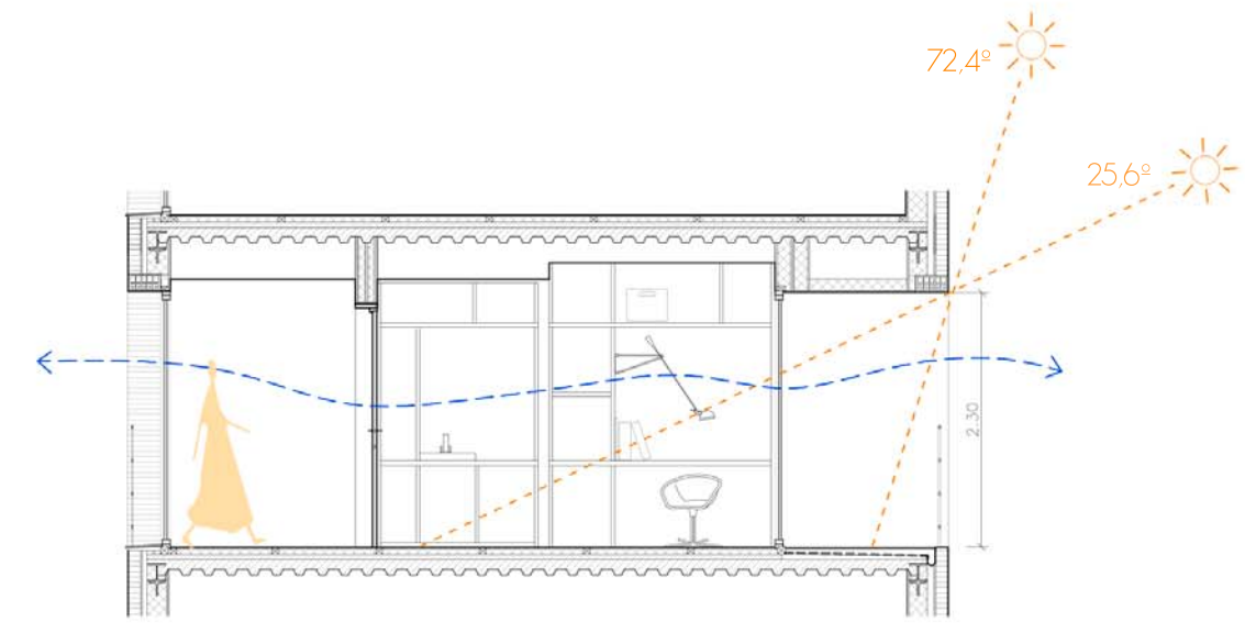
SECCIÓ F-F'
