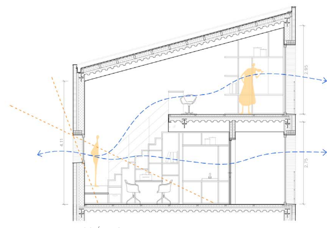
SECCIÓ B-B'
