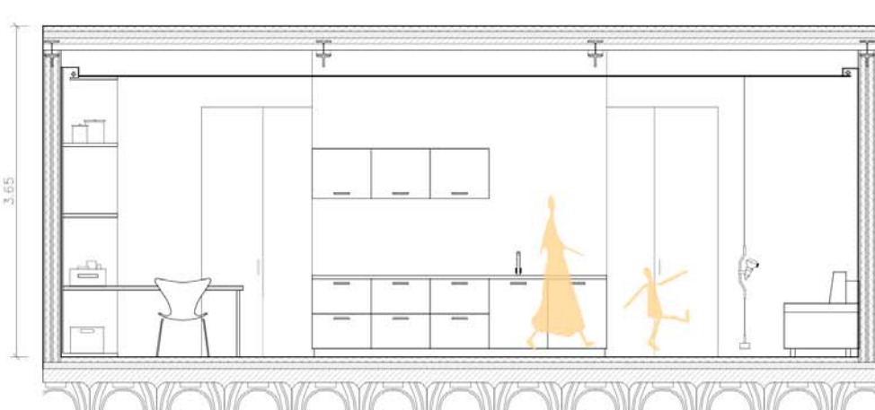
SECCIÓ L-L'
