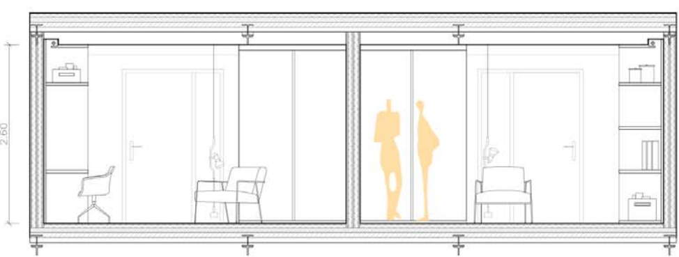
SECCIÓ H-H'
