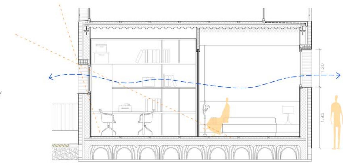
SECCIÓ J-J'
