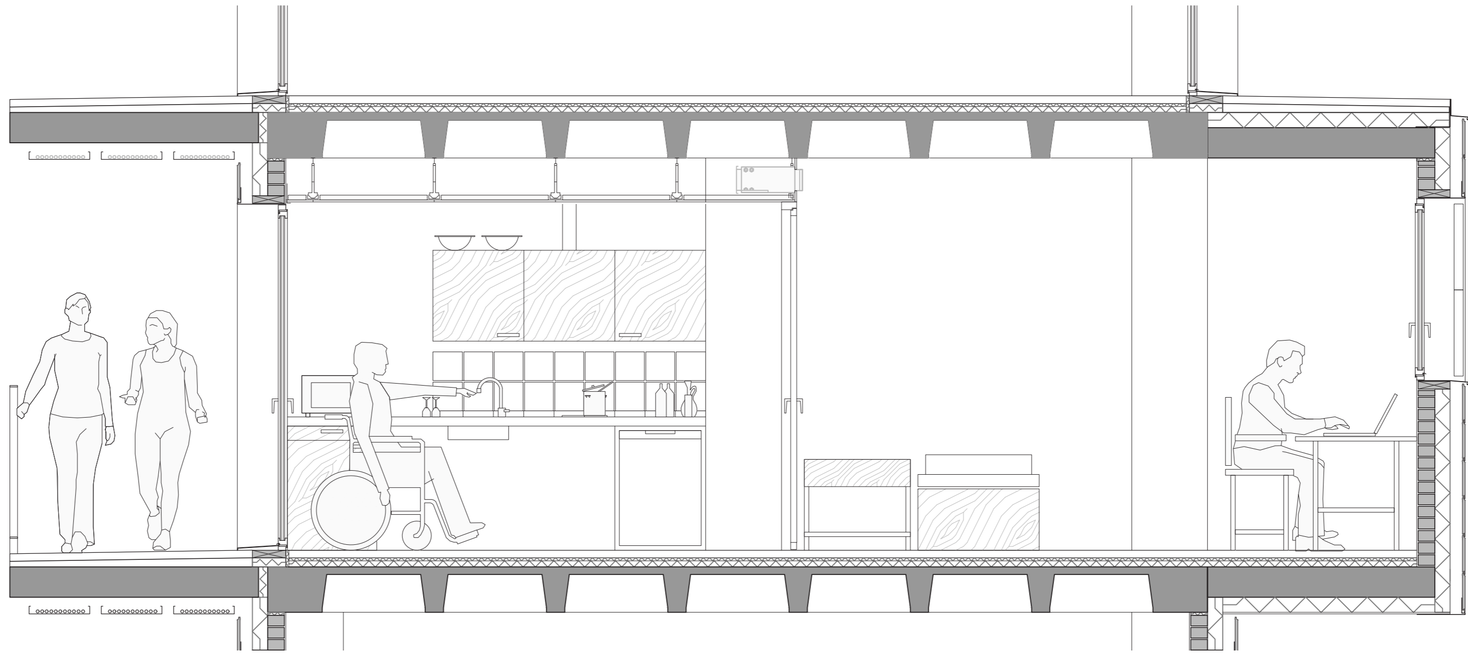
SECCIÓN E 1:25
