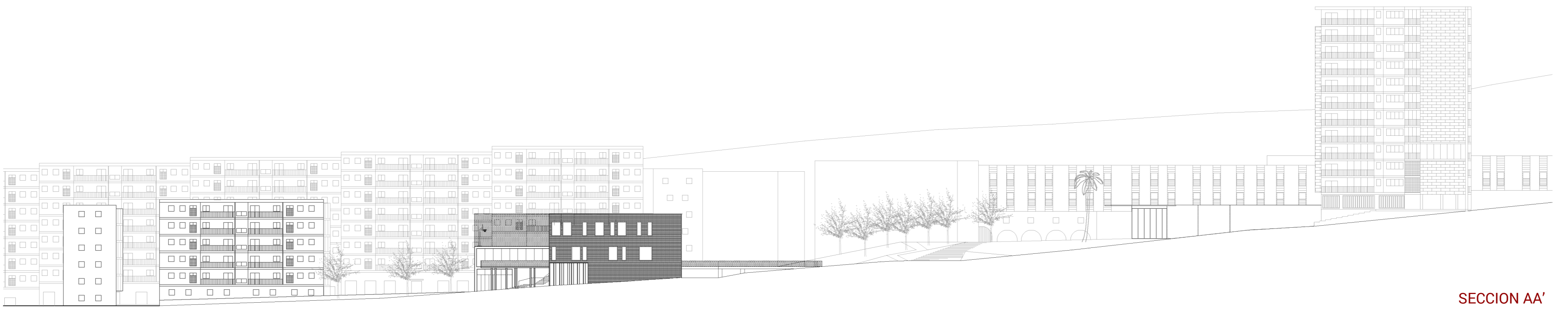
SECCION AA'
