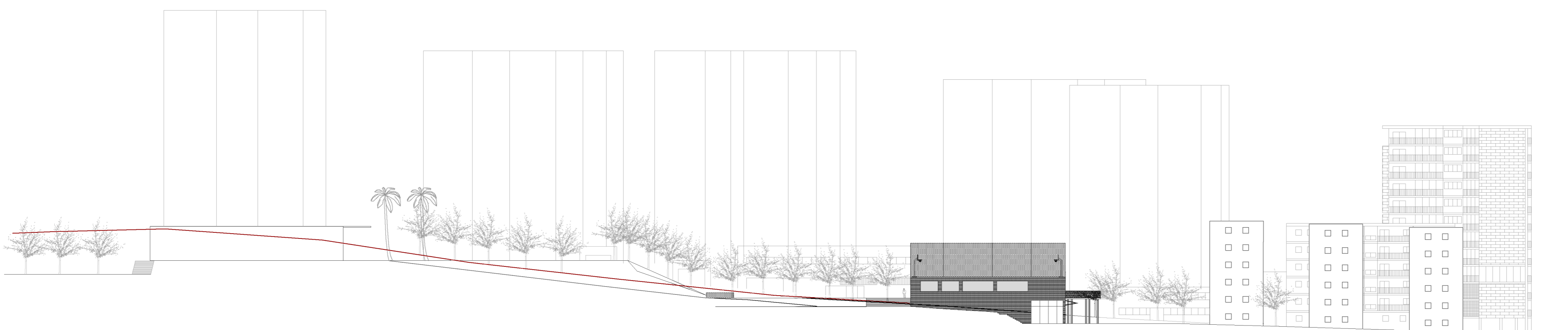
SECCION CC'
