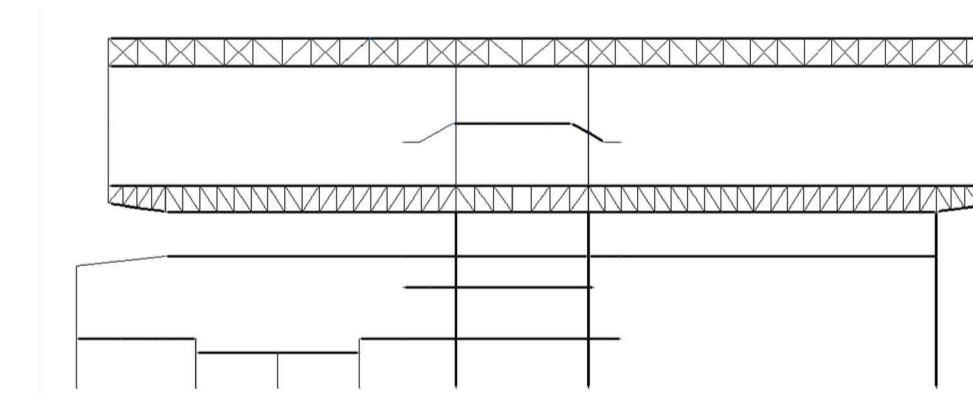
Detall de l'esquema 3D del model de càlcul - Double encavellada superior. És col·loquen perfil·s diagonals entre ambdues encavellades
