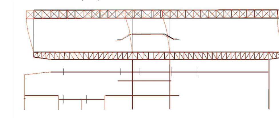
Deformada en E.L.S. en 3D (x100) Combinació de càrregues gravitatòries
