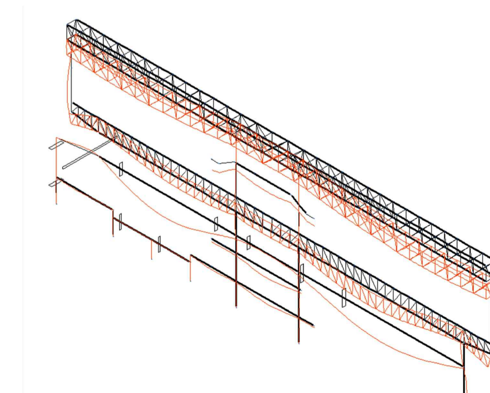
Deformada en E.L.S. en 3D (x100) Combinació de càrregues gravitatòries
