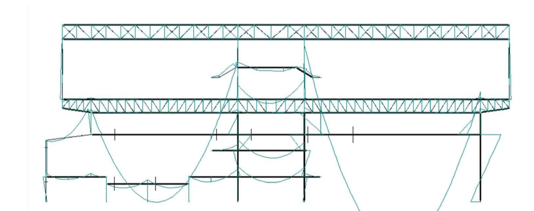
Esforsos: envoltant de moments flectors en E.L.U.
