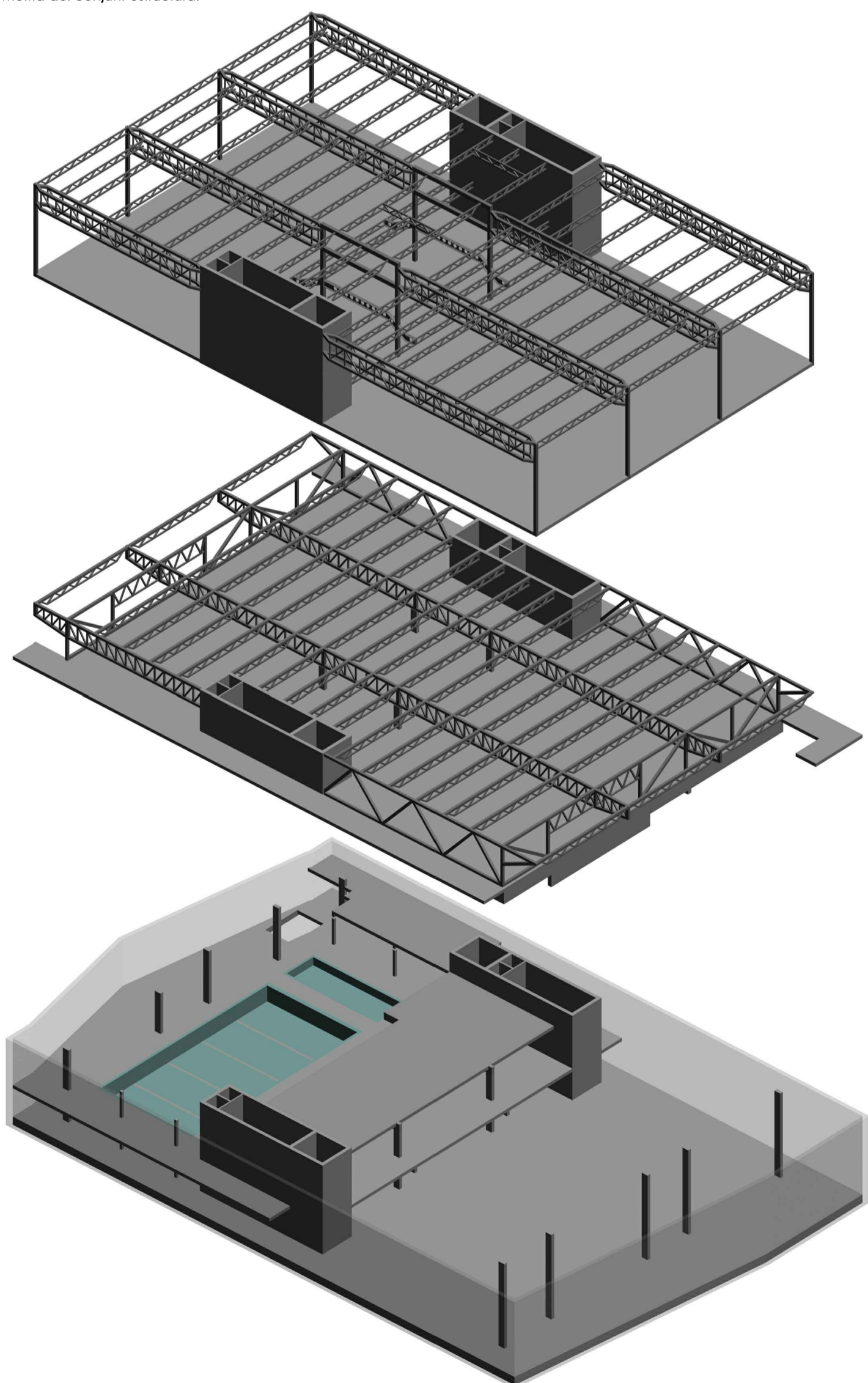
Axonometria del conjunt estructural
