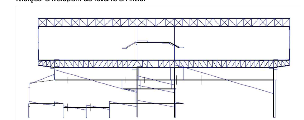
Esforsos: envoltant de tallants en E.L.U.
