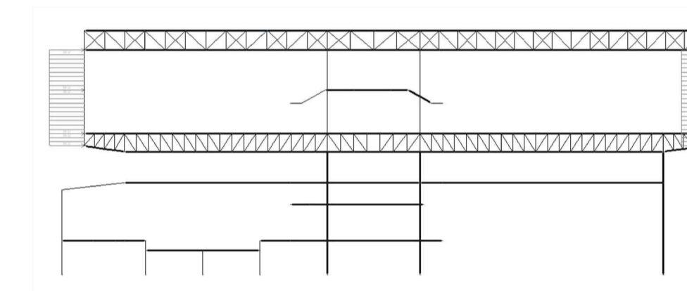
Deformada en E.L.S. (x100) Combinació de càrregues gravitatòries (G + Q1 + Q2 + ...)
