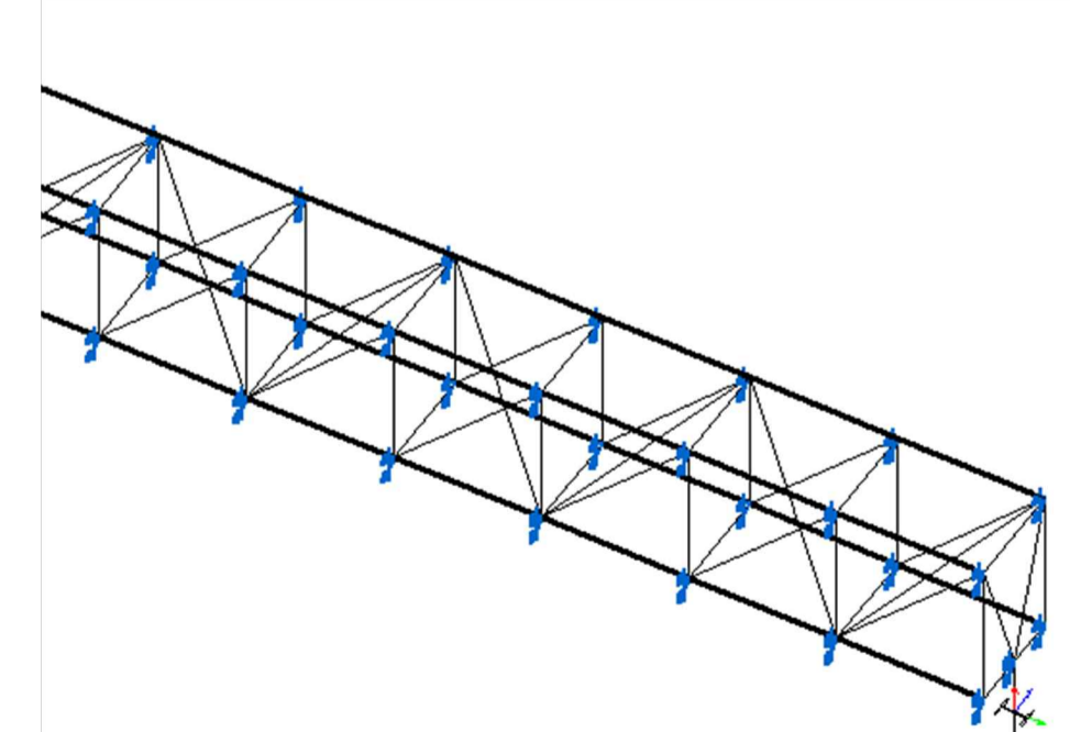
Detall de l'esquema 3D del model de càlcul - Double encavellada superior. És col·loquen perfil·s diagonals entre ambdues encavellades
