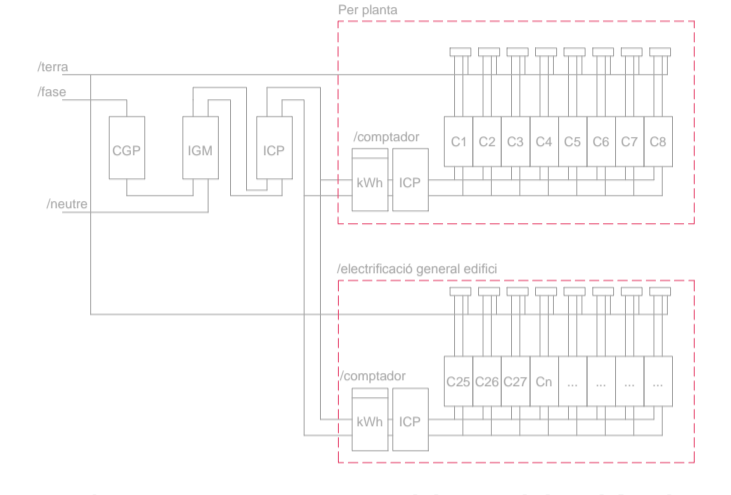
/esquema general instal·lació electricitat
