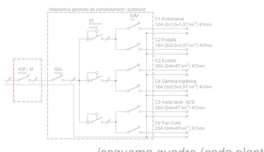
/esquema quadre (cada planta)
