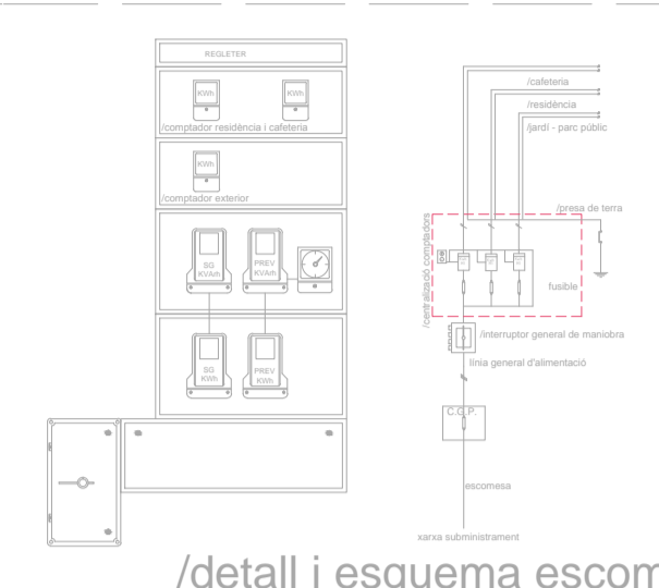
/detall i esquema escomesa general
