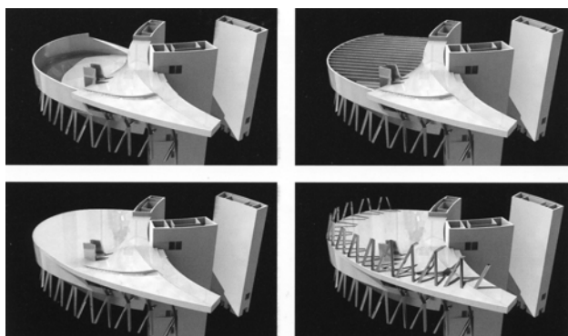
Figura 9.- Diagramas de solución estructural del museo para la Mercedes-Benz [3]
