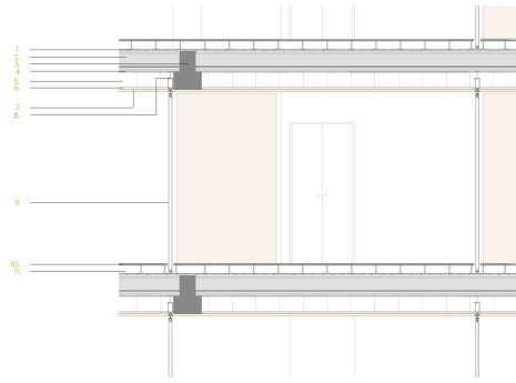
DETALL ACABATS INTERIORS PEÇES _E 1/50
