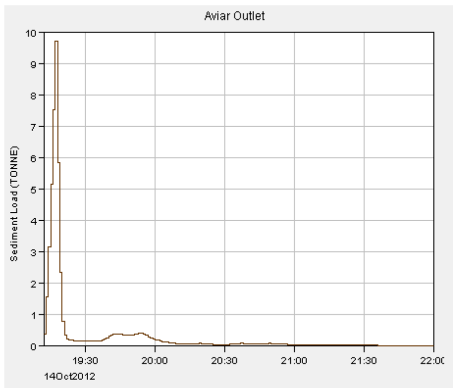
Il·lustració 18. Sedimentograma Episodi 9.
