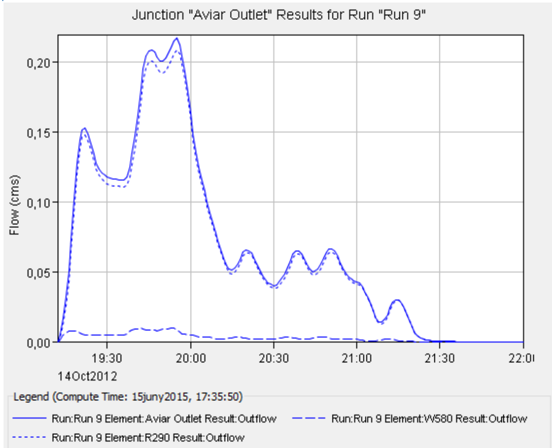
Il·lustració 17. Hidrograma Episodi 9.
