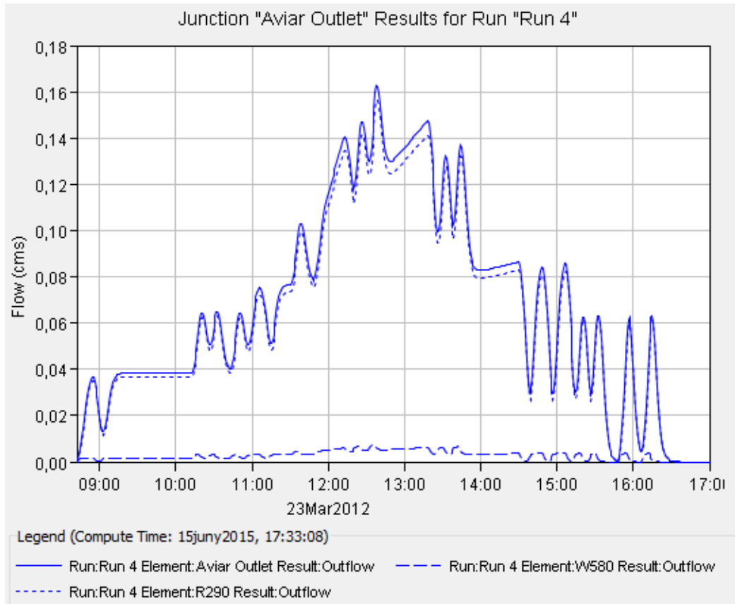
Il·lustració 7. Hidrograma Episodi 4.
