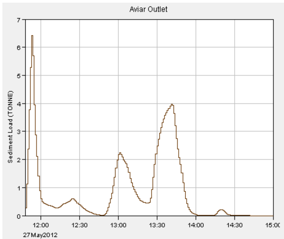
Il·lustració 14. Sedimentograma Episodi 7.
