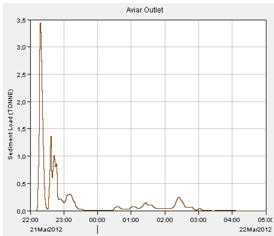
Il·lustració 4. Sedimentograma Episodi 2.
