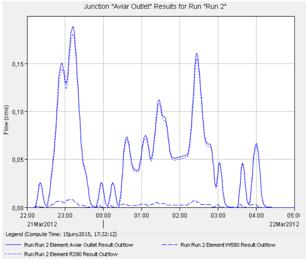
Il·lustració 3. Hidrograma Episodi 2.
