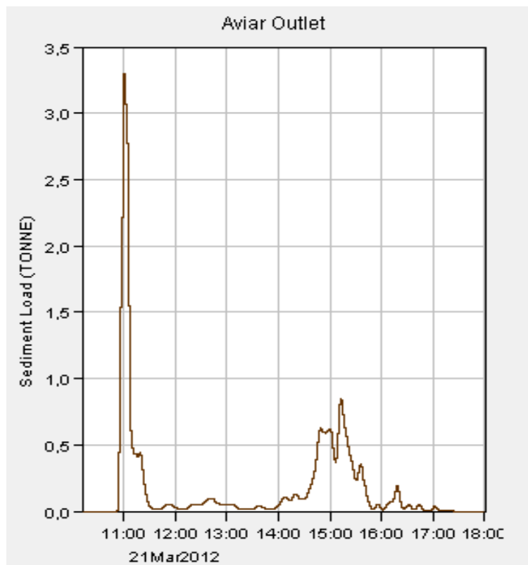
Il·lustració 2. Sedimentograma Episodi 1.
