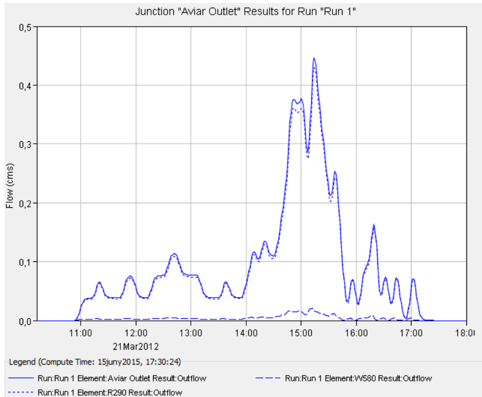
Il·lustració 1. Hidrograma Episodi 1.
