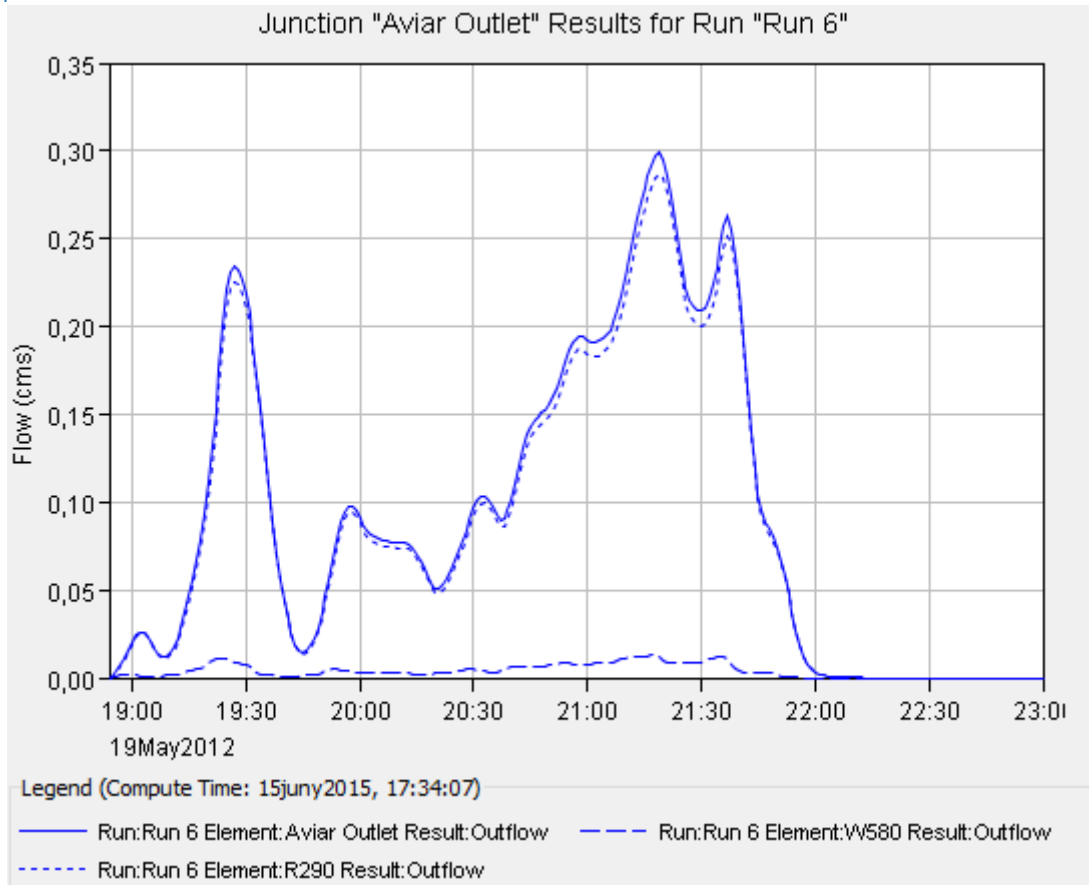
Il·lustració 11. Hidrograma Episodi 6.
