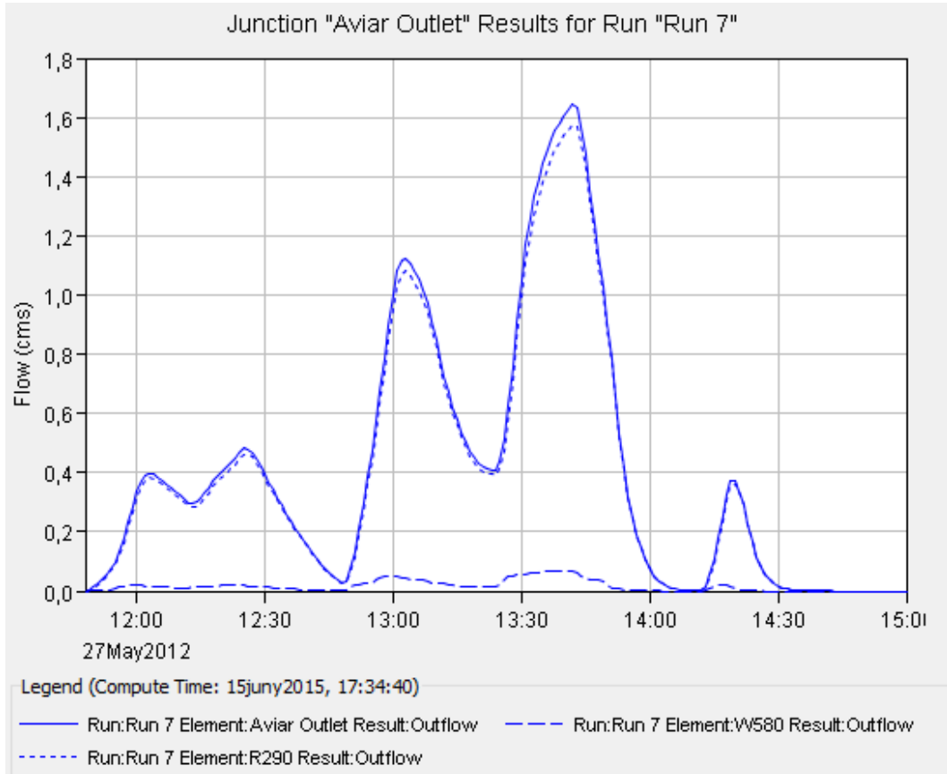
Il·lustració 13. Hidrograma Episodi 7.
