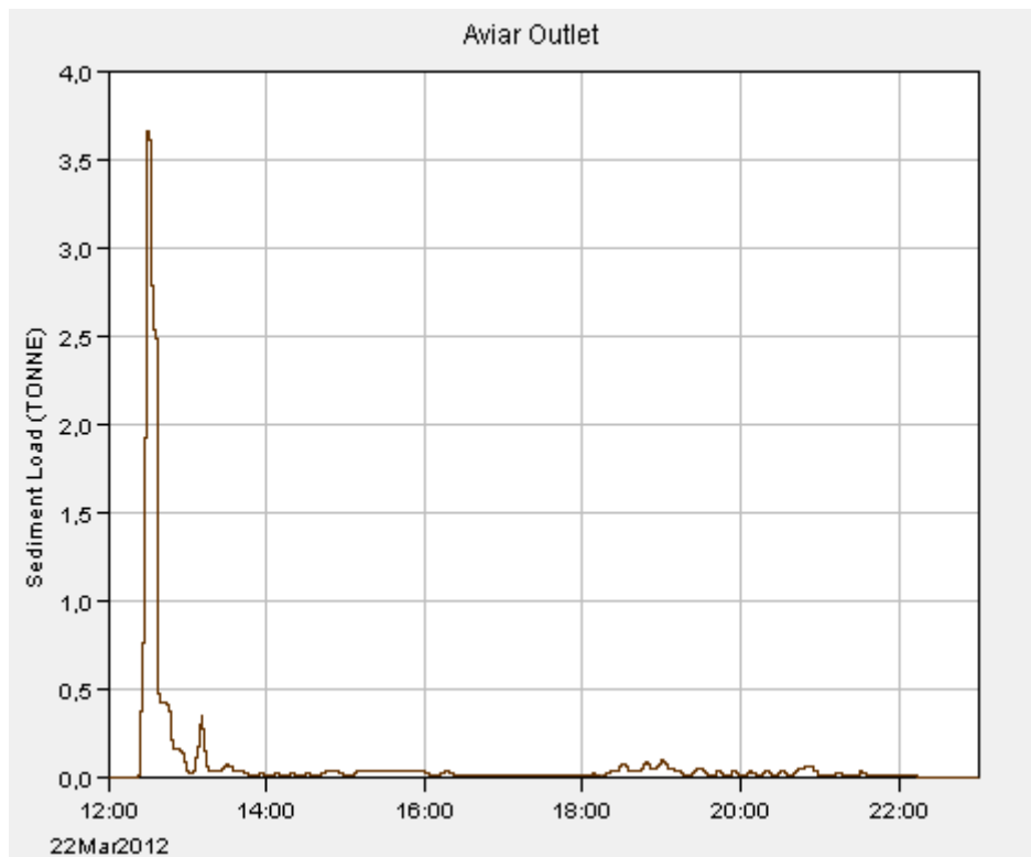
Il·lustració 6. Sedimentograma Episodi 3.
