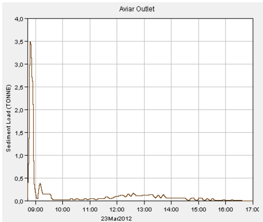
Il·lustració 8. Sedimentograma Episodi 4.
