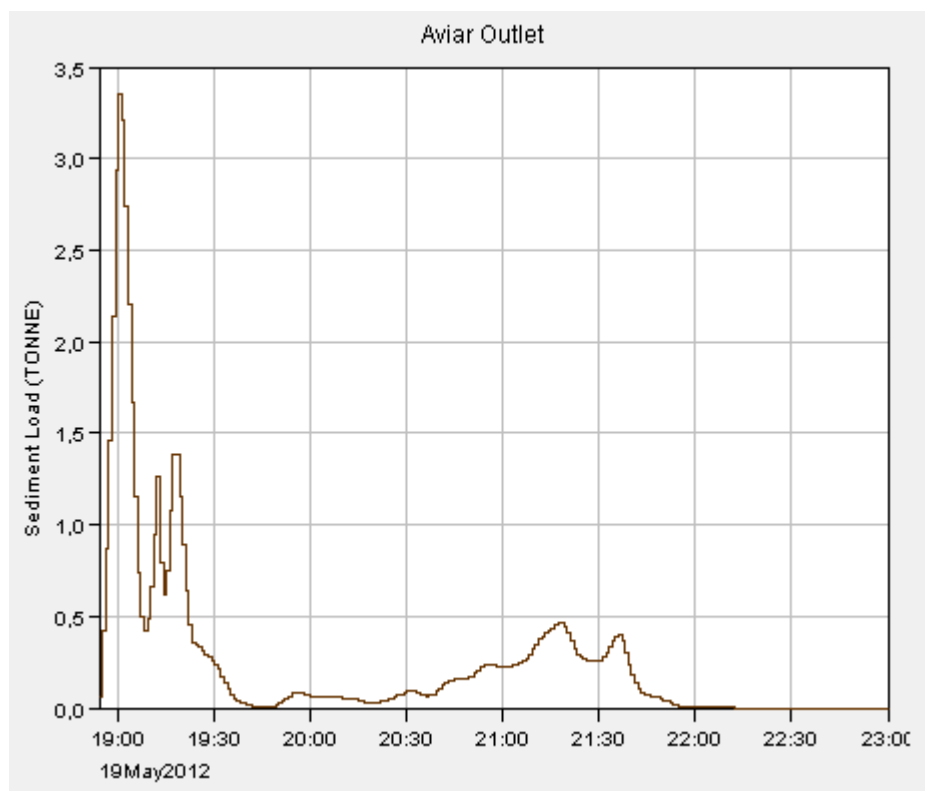
Il·lustració 12. Sedimentograma Episodi 6.
