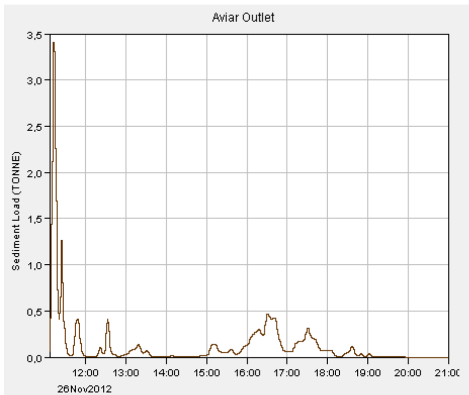
Il·lustració 24. Sedimentograma Episodi 12.
