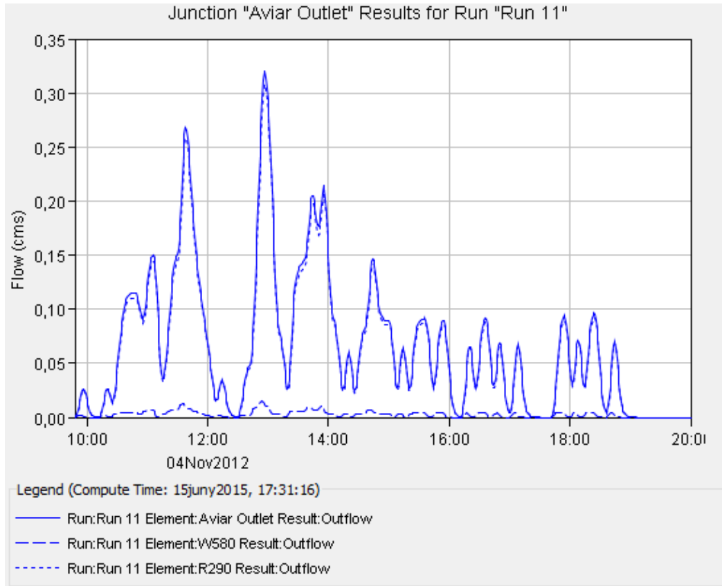
Il·lustració 21. Hidrograma Episodi 11.
