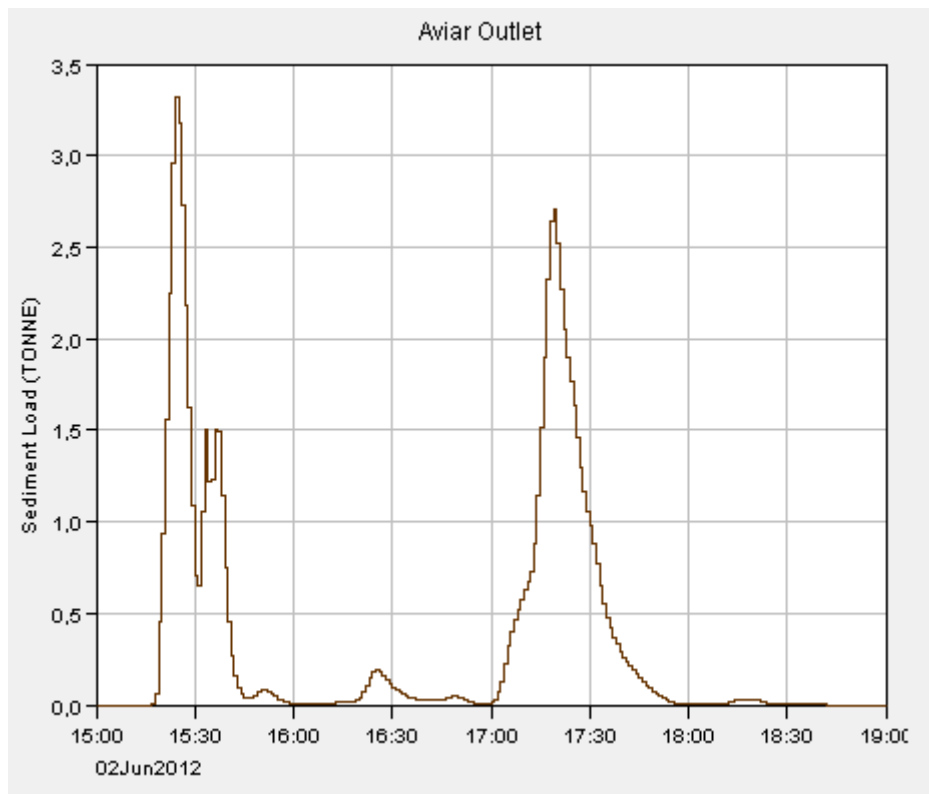
Il·lustració 16. Sedimentograma Episodi 8.
