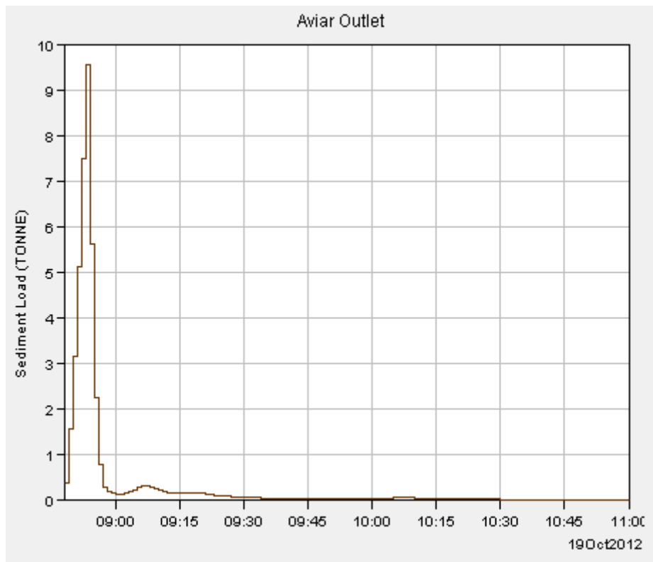
Il·lustració 20. Sedimentograma Episodi 10.
