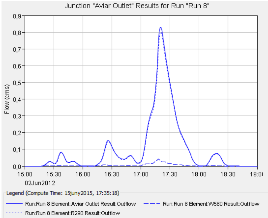
Il·lustració 15. Hidrograma Episodi 8.
