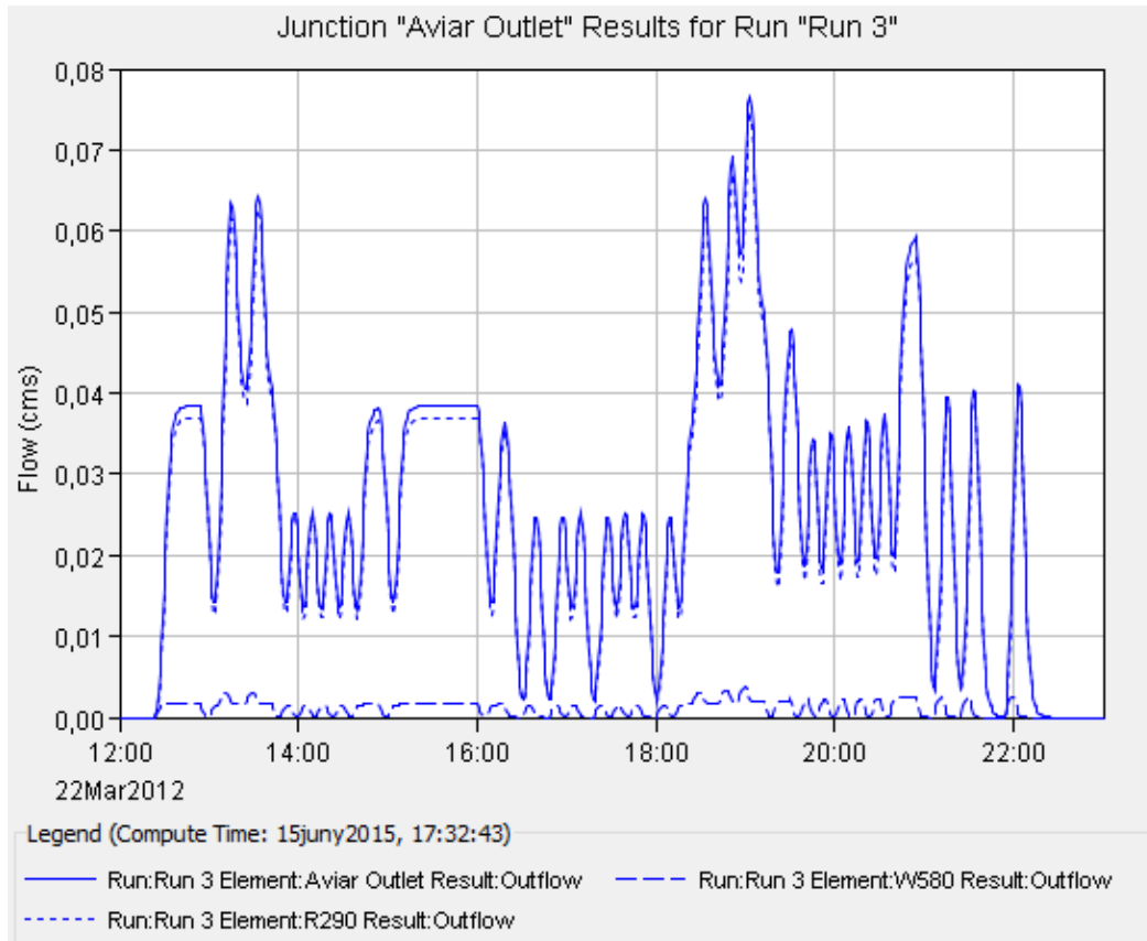
Il·lustració 5. Hidrograma Episodi 3.
