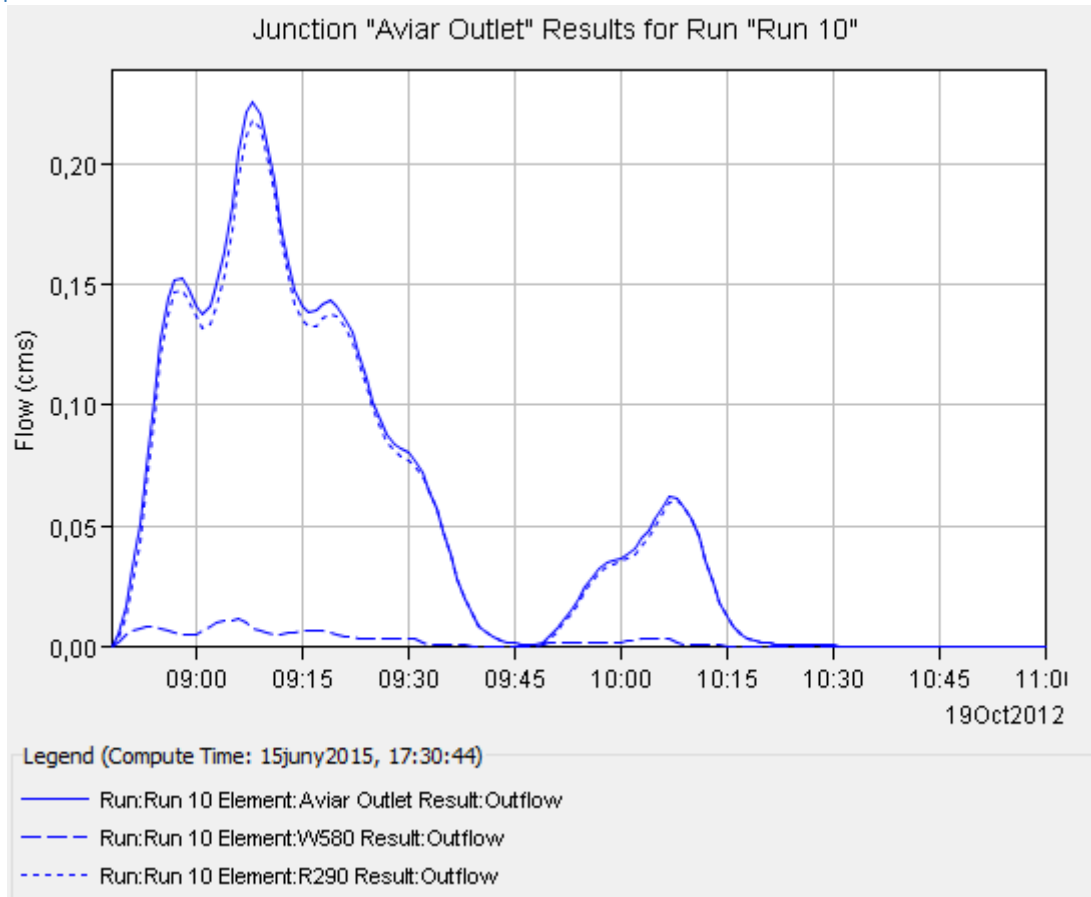
Il·lustració 19. Hidrograma Episodi 10.
