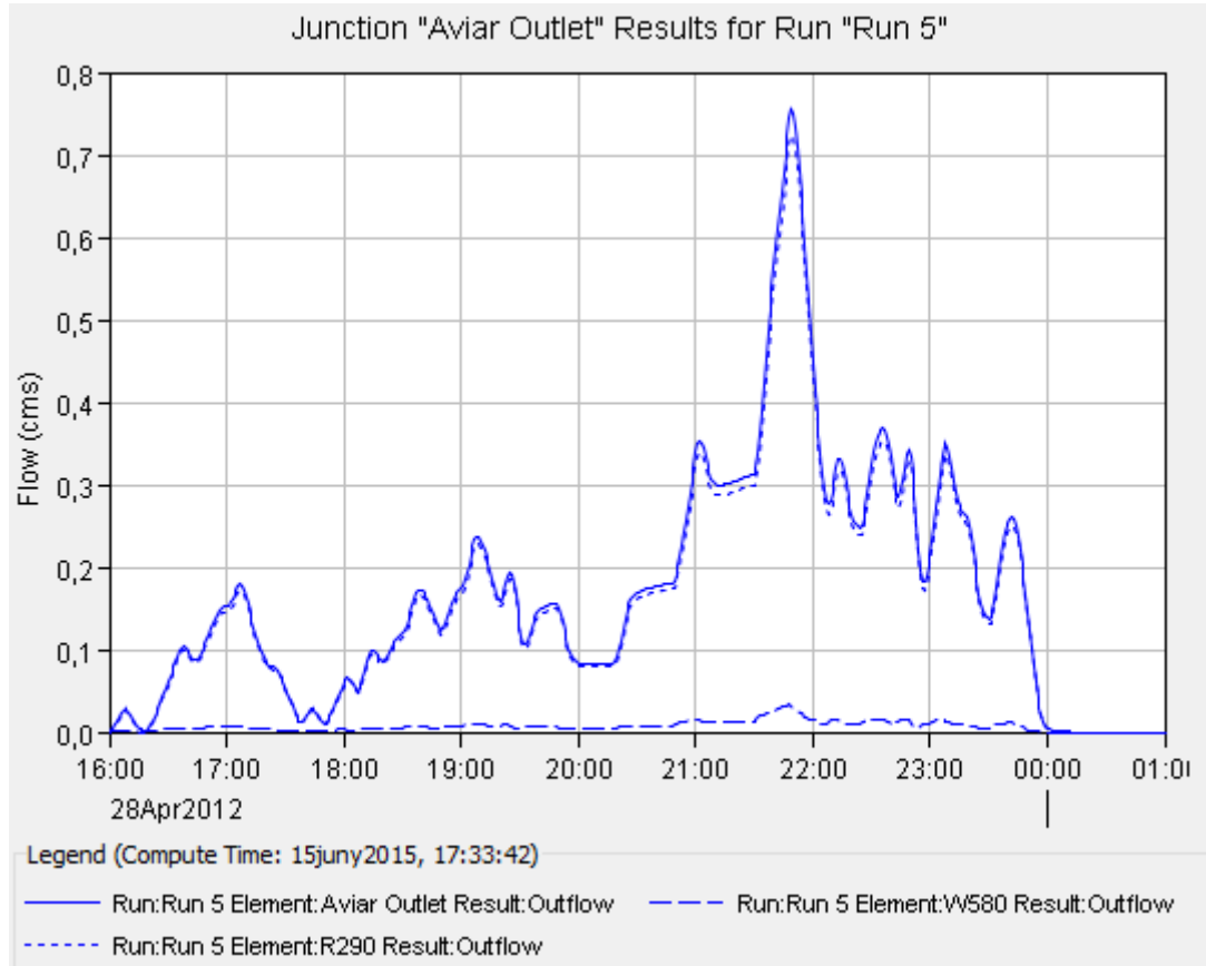
Il·lustració 9. Hidrograma Episodi 5.
