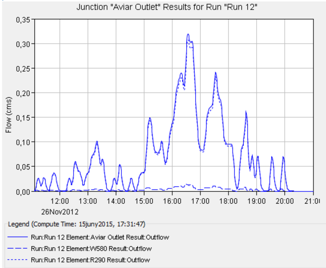
Il·lustració 23. Hidrograma Episodi 12.
