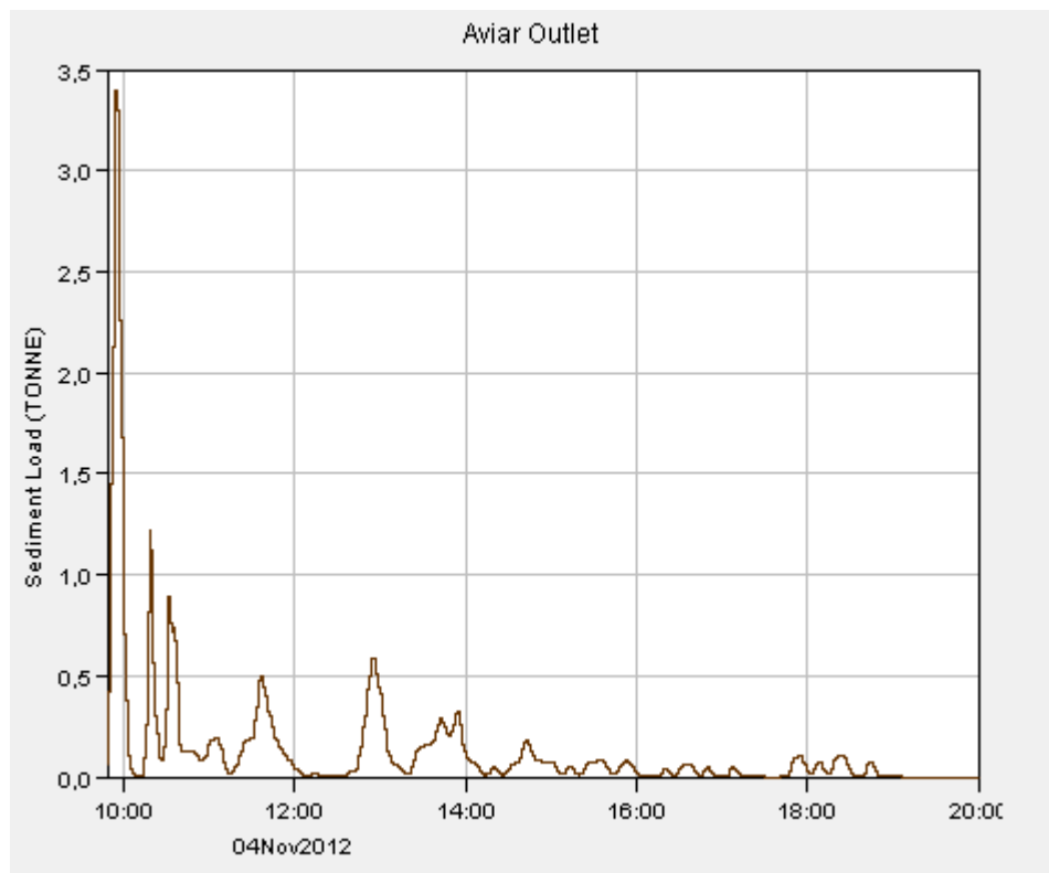
Il·lustració 22. Sedimentograma Episodi 11.
