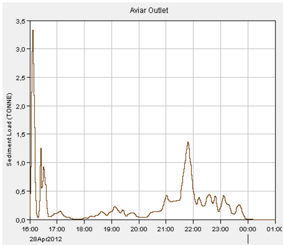
Il·lustració 10. Sedimentograma Episodi 5.
