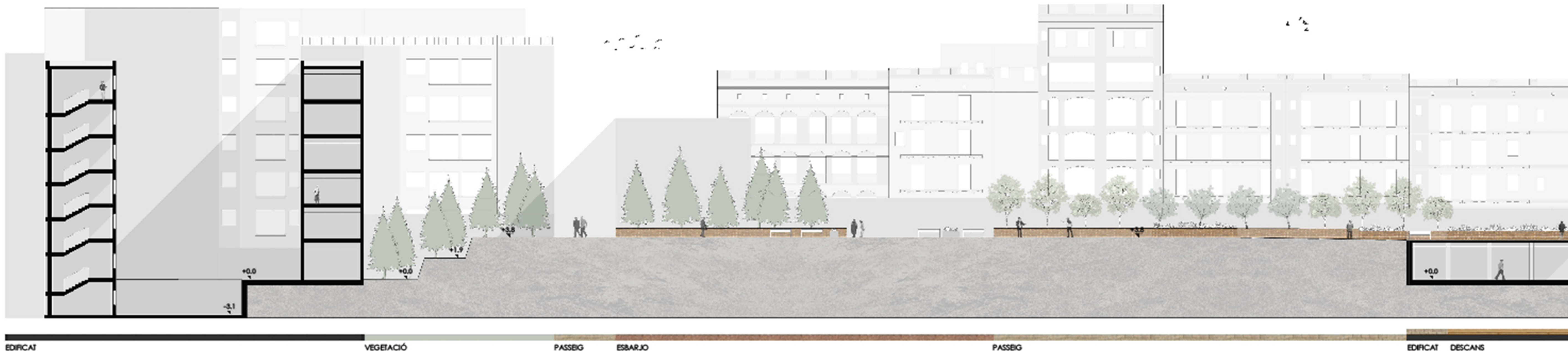
S1. SECCIÓ TRANSVERSAL SUD-OEST
