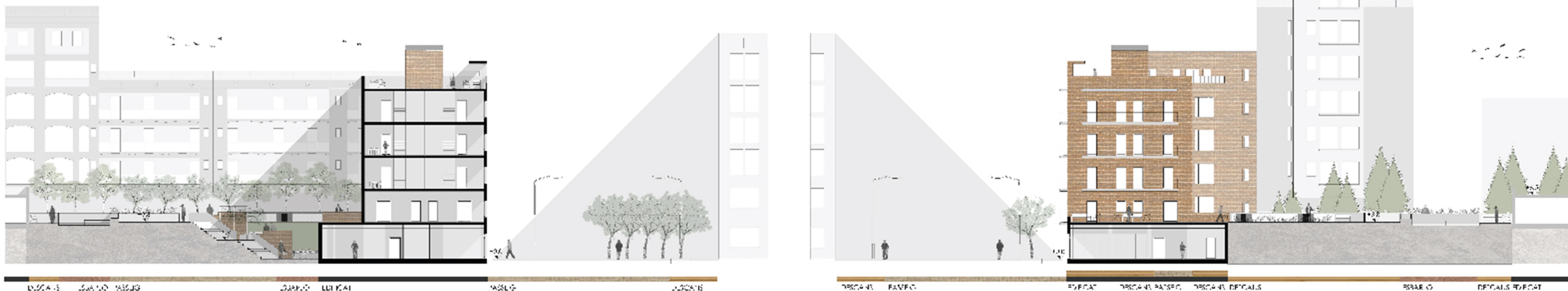
S3. SECCIÓ LONGITUDINAL EST-OEST
