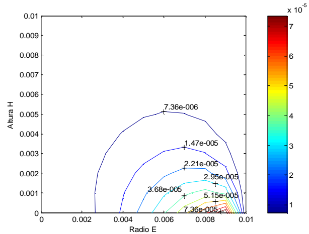
Figura 3. Función circulación ( \Gamma ) para Re=3 \times 10^4 y factor de forma 1
