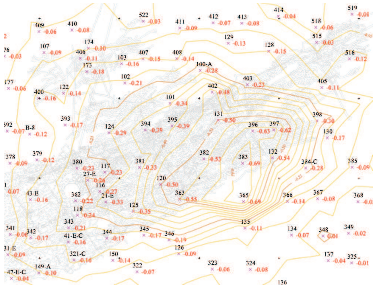
Figura 1. Mapa vectorial de isolíneas de hundimiento 2011-2013 en zona de máxima subsidencia de Cabanasses
