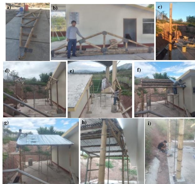
Figura 4. Fases de construcción del prototipo de Bambú a escala real y la colocación de los sistemas de medición. a) montaje de celosía de bambú, b) Conexiones en la celosía de bambú, c) izado de las columnas de bambú, d) y e) colocación de celosías del techo del prototipo de vivienda, f) colocación de las correas de bambú y cobertura de calamina, g) Verificación de niveles de la cobertura, h) Colocación de sistemas de medición con varillas de acero corrugado y i) colocación de los sistemas de medición.
