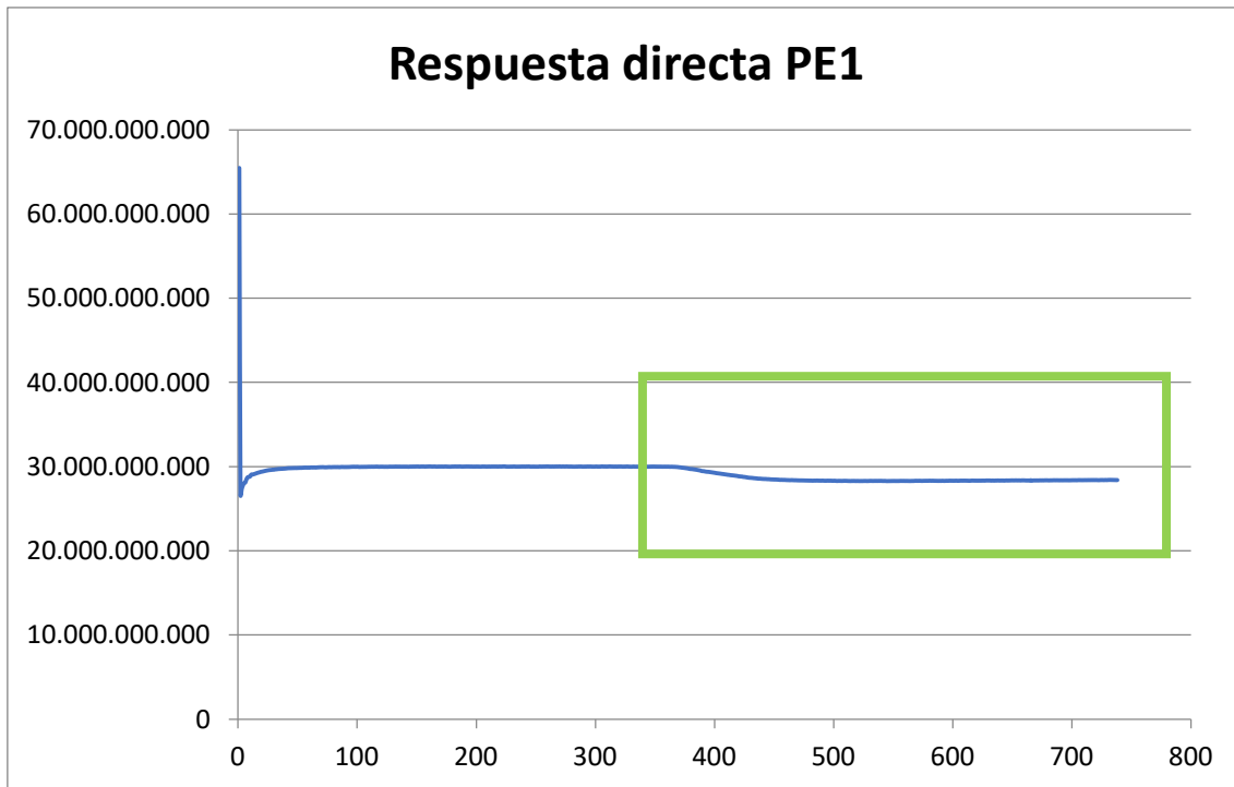
Gráfico 1 Respuesta directa del ensayo PE1
