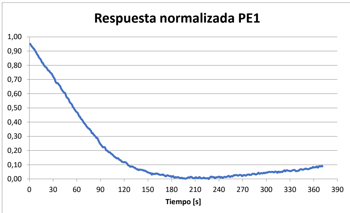
Gráfico 2 Respuesta normalizada del ensayo PE1
