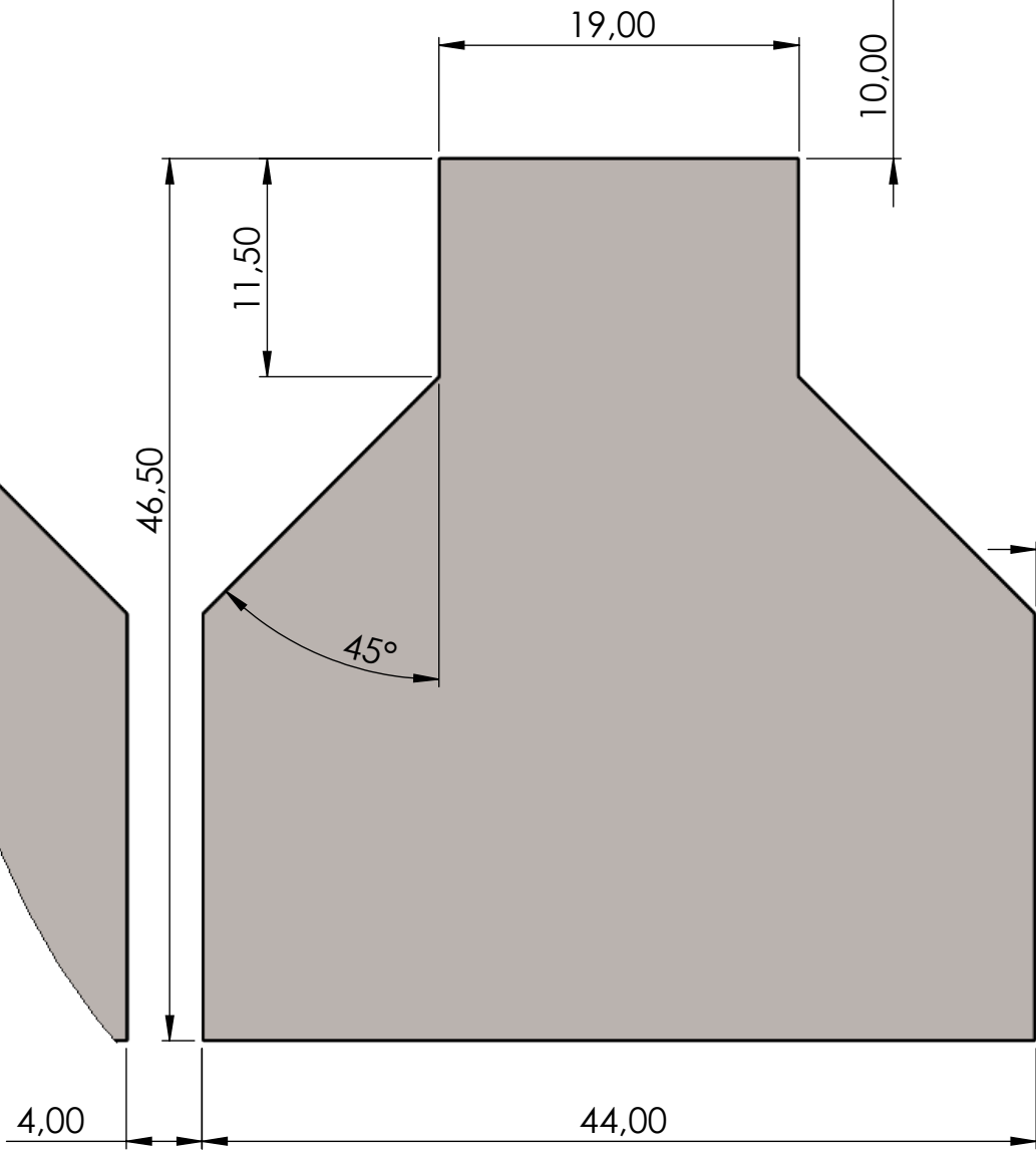
DETALLE A ESCALA 2.5 : 1
