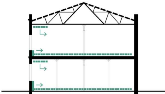
Nova xapa de compressió superior amb connexió a forjats
