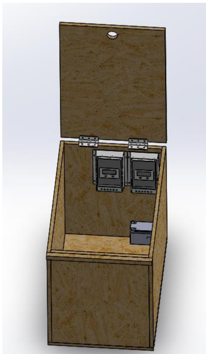
Il·lustració 5: Col·locació específica instal·lació elèctrica a l'armari esquerre
