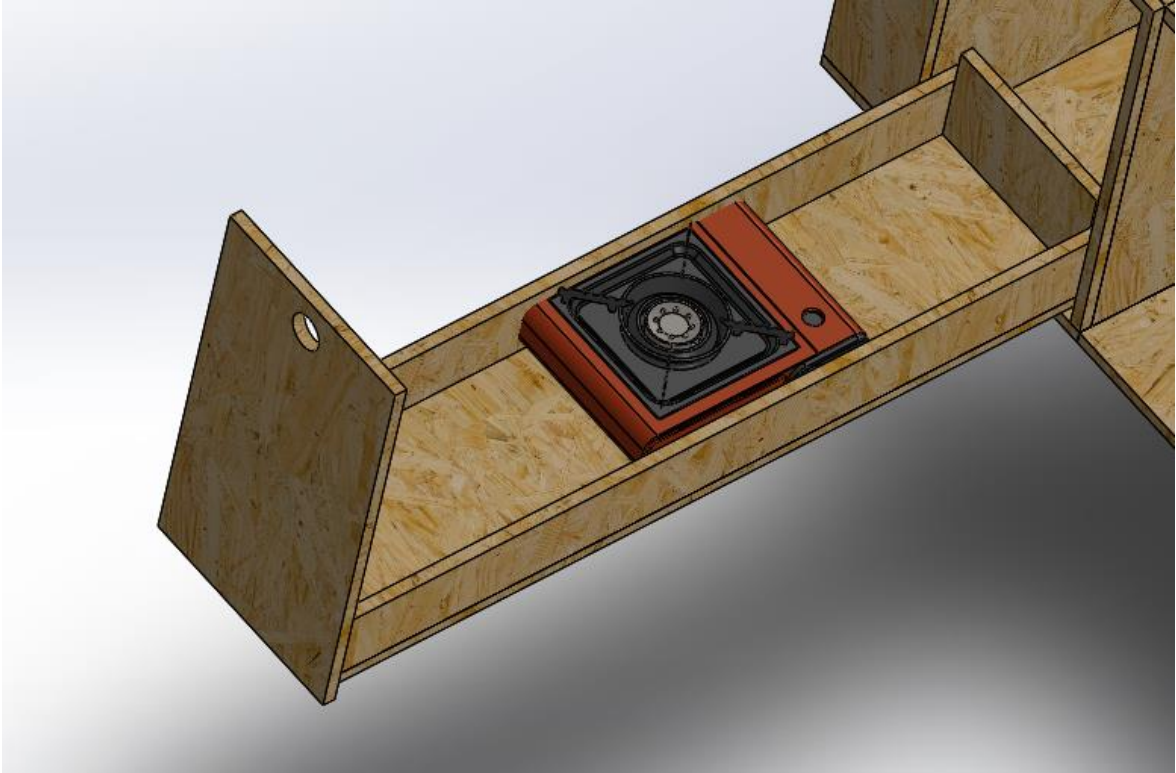
Il·lustració 2: Col·locació específica fogó al banc esquerre.
