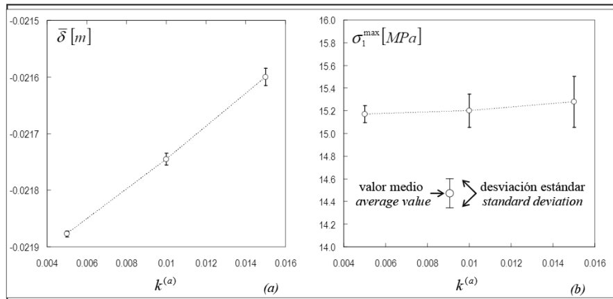
Figura 7. Viga de tres puntos: (a) deflexión en la mitad de la luz promedio y su desviación estándar, (b) esfuerzo principal máximo a tensión promedio y su desviación estándar.
