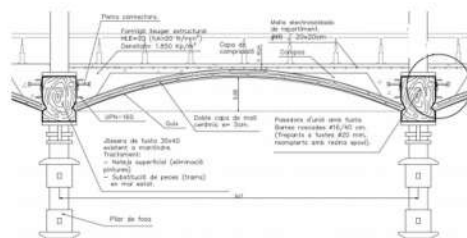
Secció de la resolució per al cobriment de l'estructura
