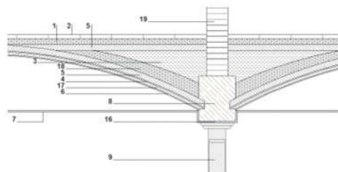
Secció tipus del sostre en el toberaner amb un pilar de fosa
