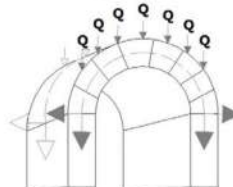
Esquema del descens de càrregues en una volta de canó
