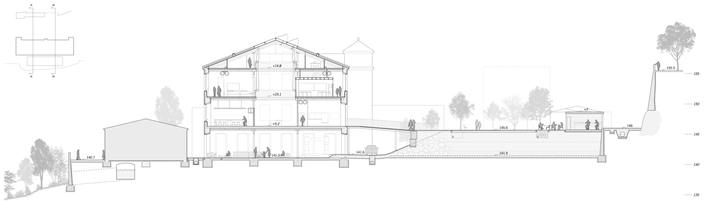
Secció A
