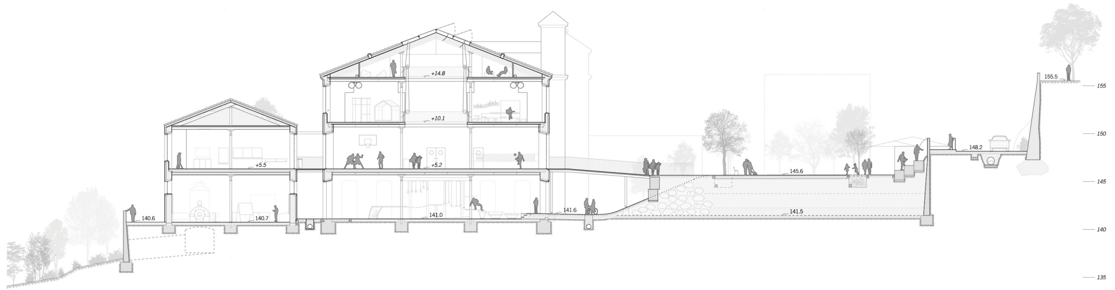
Secció B
