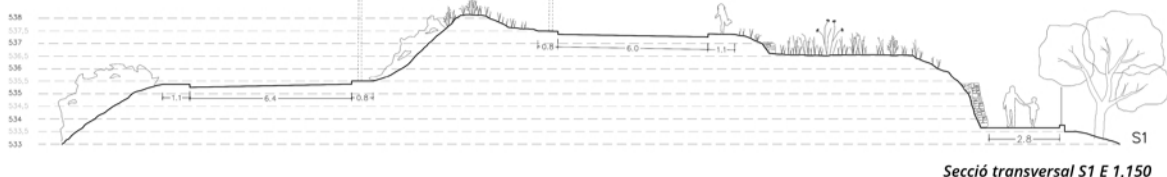
Secció transversal S1 E 1.150
