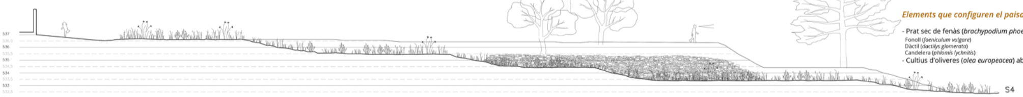
Secció longitudinal S4 E 1.150
