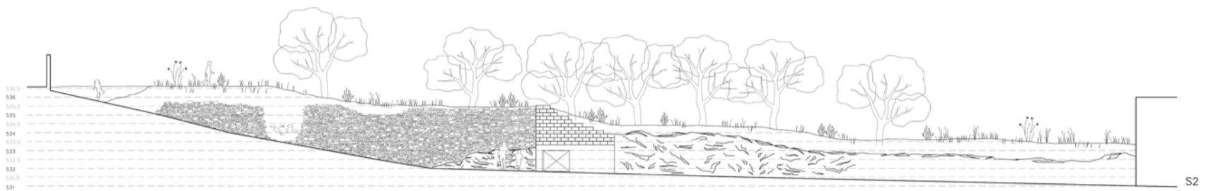
Secció longitudinal S2 E 1.150
