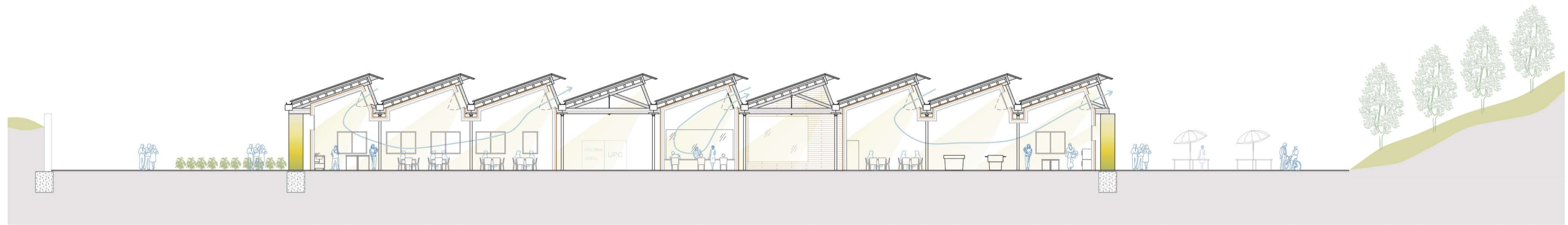
Sección zonas comunes | Escala 1:100
