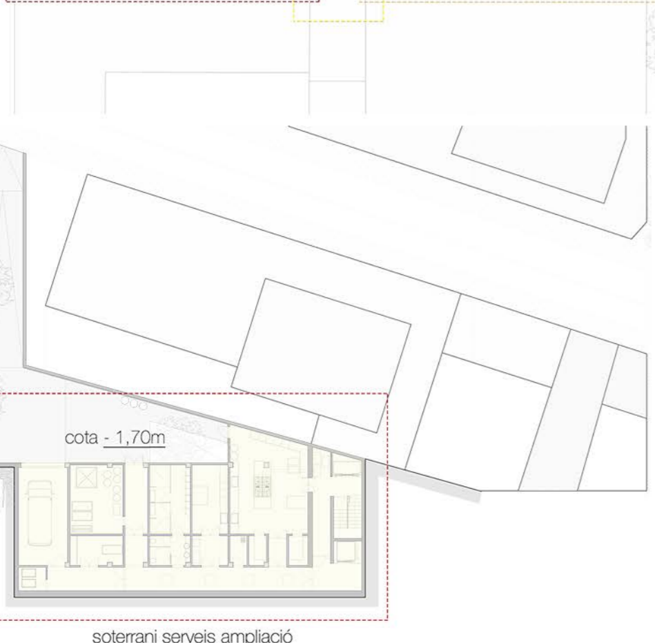
estratègia de cotes i ampliació e1/300
