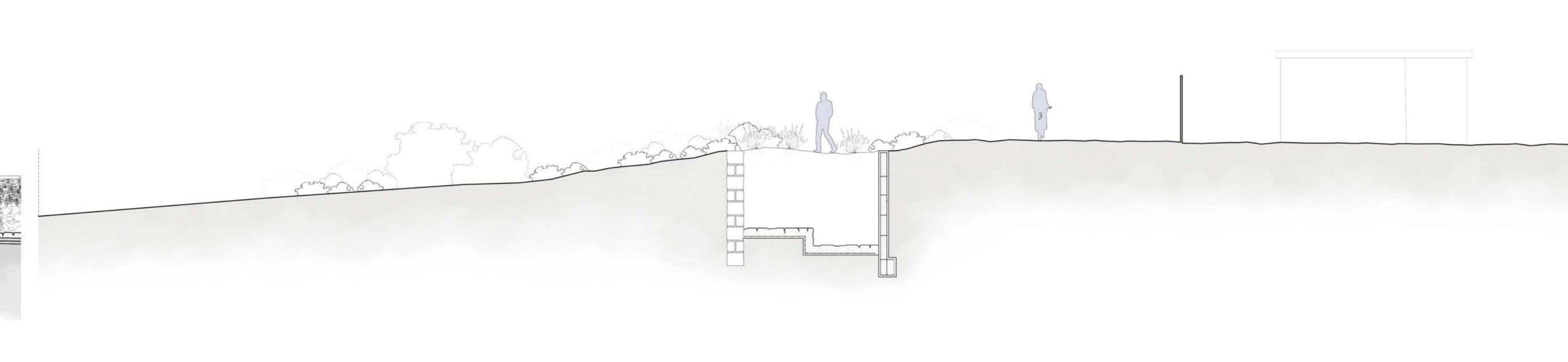
SECCIÓN 8 CANAL - SALINERA
