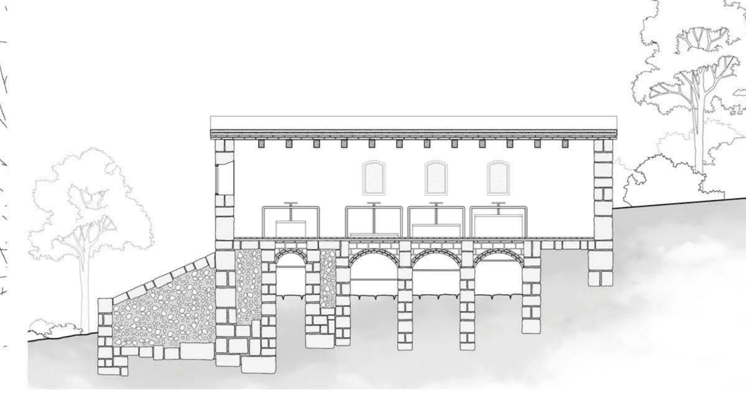
SECCIÓN 1 ESCLUSA DE L'ARANYÓ
