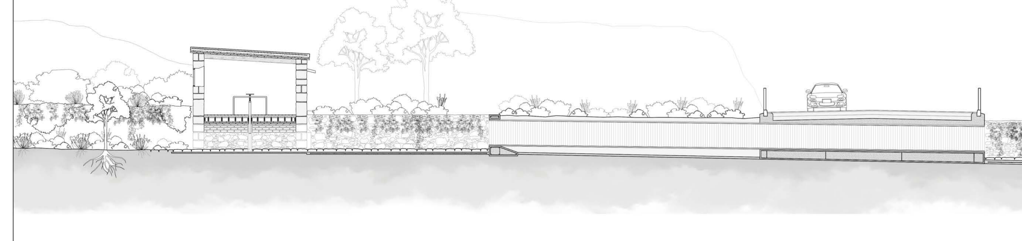
SECCIÓN 4 ESCLUSA - CARRETERA NUEVA
