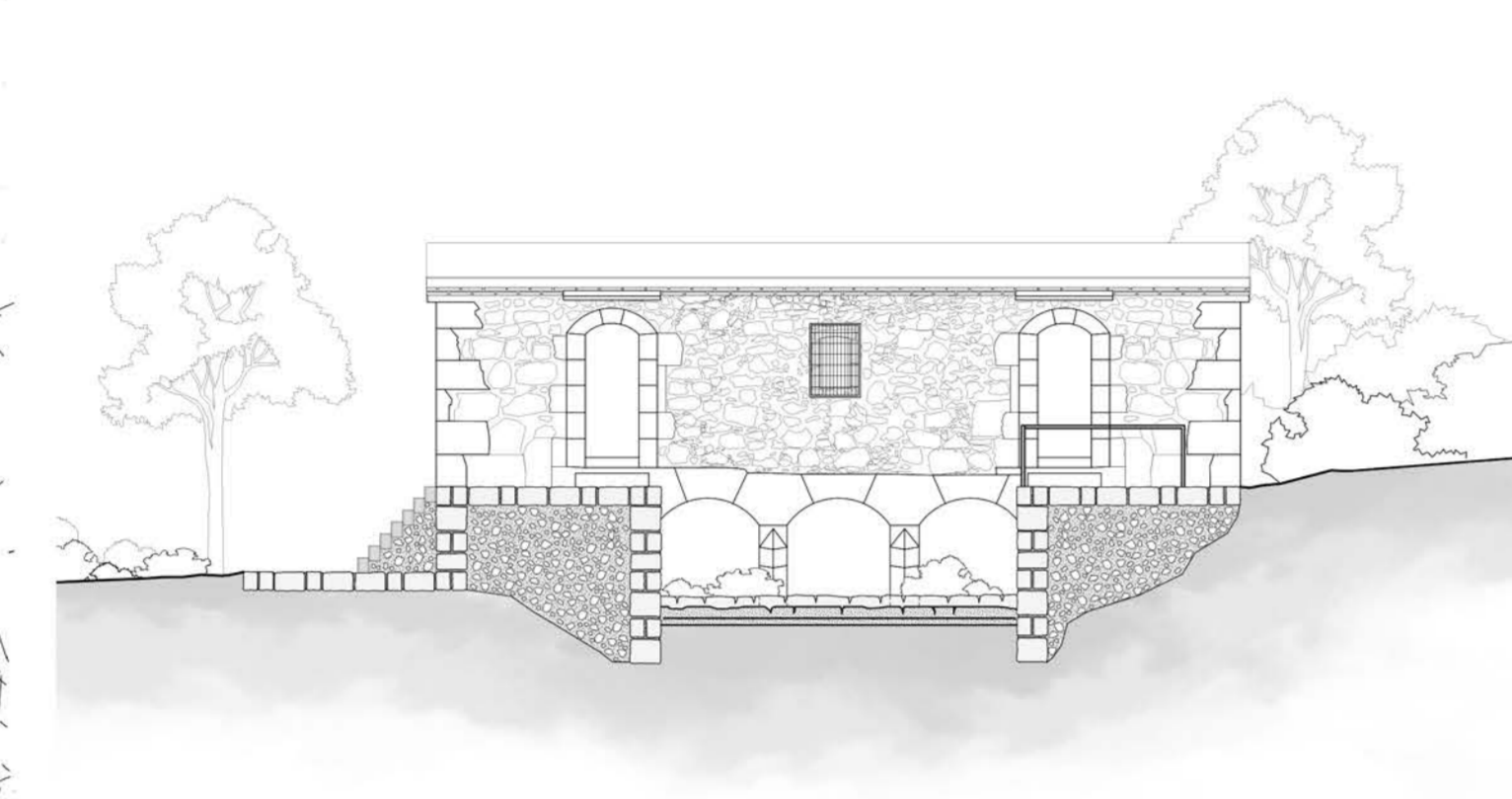
SECCIÓN 2 PATIO ESCLUSA DE L'ARANYÓ
