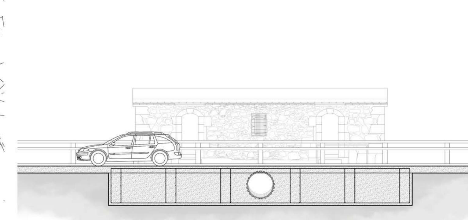
SECCIÓN 3 CARRETERA NUEVA
