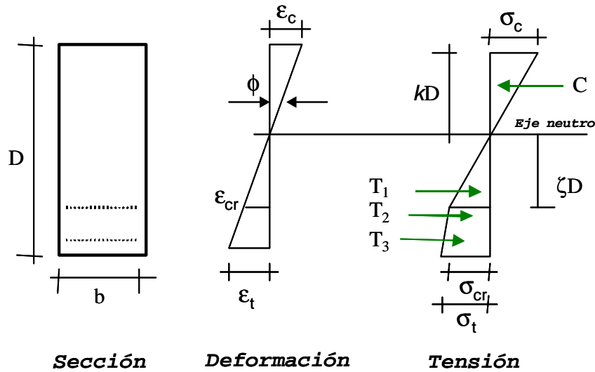
Figura 6. Distribución de deformaciones y de tensiones, cuando sólo el lado a tracción sale del intervalo elástico.
