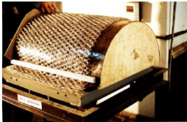
Fotografía 9. Refuerzo sobre formaleta en madera para tanque cilíndrico [Bedoya 96]
