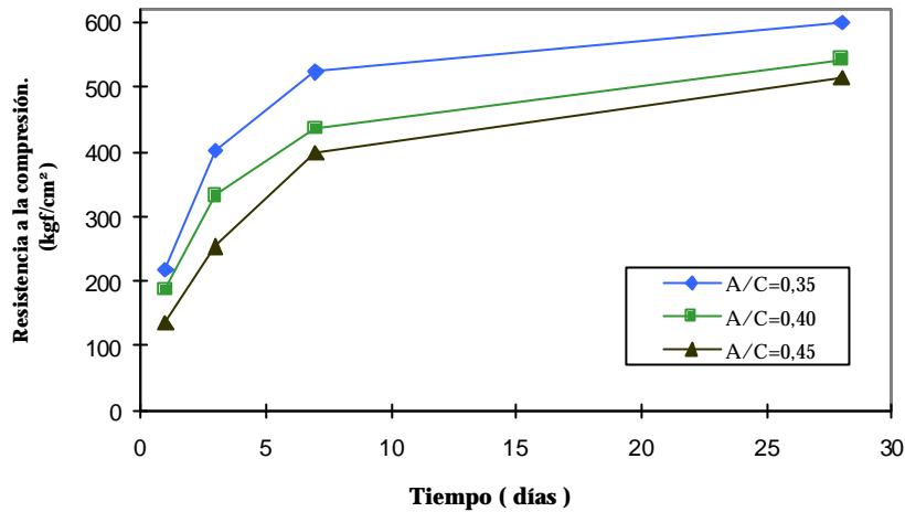
Figura 2. Efecto de la relación agua – cemento en la resistencia [Bedoya 96].
