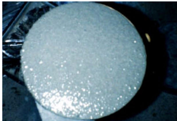
Fotografía 8. Consistencia no deseada del mortero para ferrocemento [Bedoya 96].
