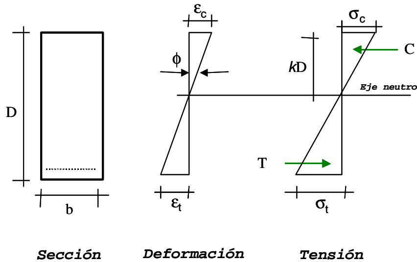
Figura 5. Distribución de deformaciones y tensiones en el intervalo elástico
