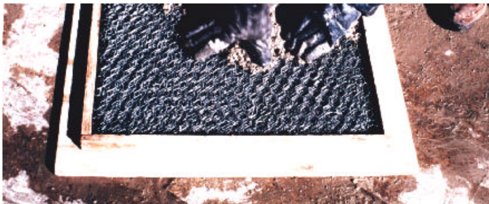
Fotografía 3. Refuerzo tipo malla hexagonal [Bedoya 96].
