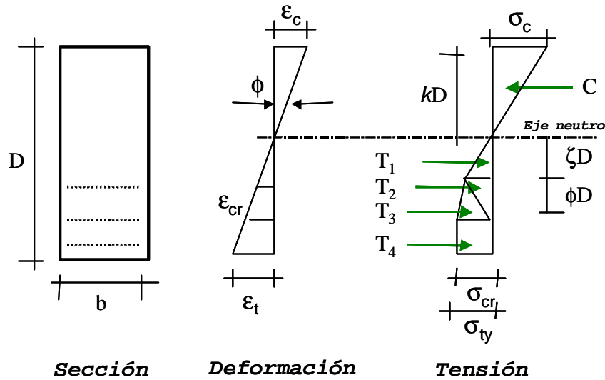
Figura 8. Distribución de deformaciones y de tensiones cuando el refuerzo está cediendo y el mortero a compresión está en el intervalo elástico.
