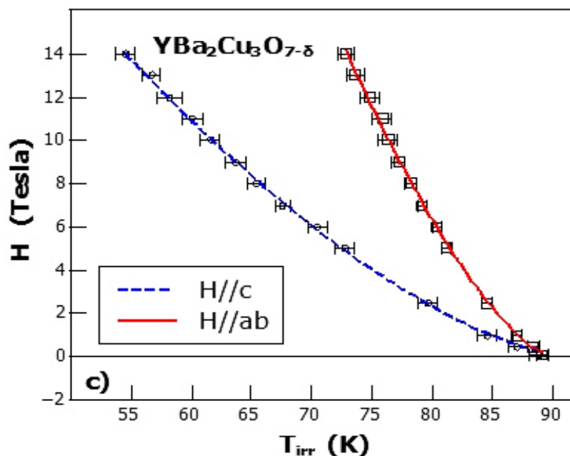
Figura 2 Comportamento da linha de Irreversibilidade magnética com campo aplicado ao longo do plano ab e do eixo c .
