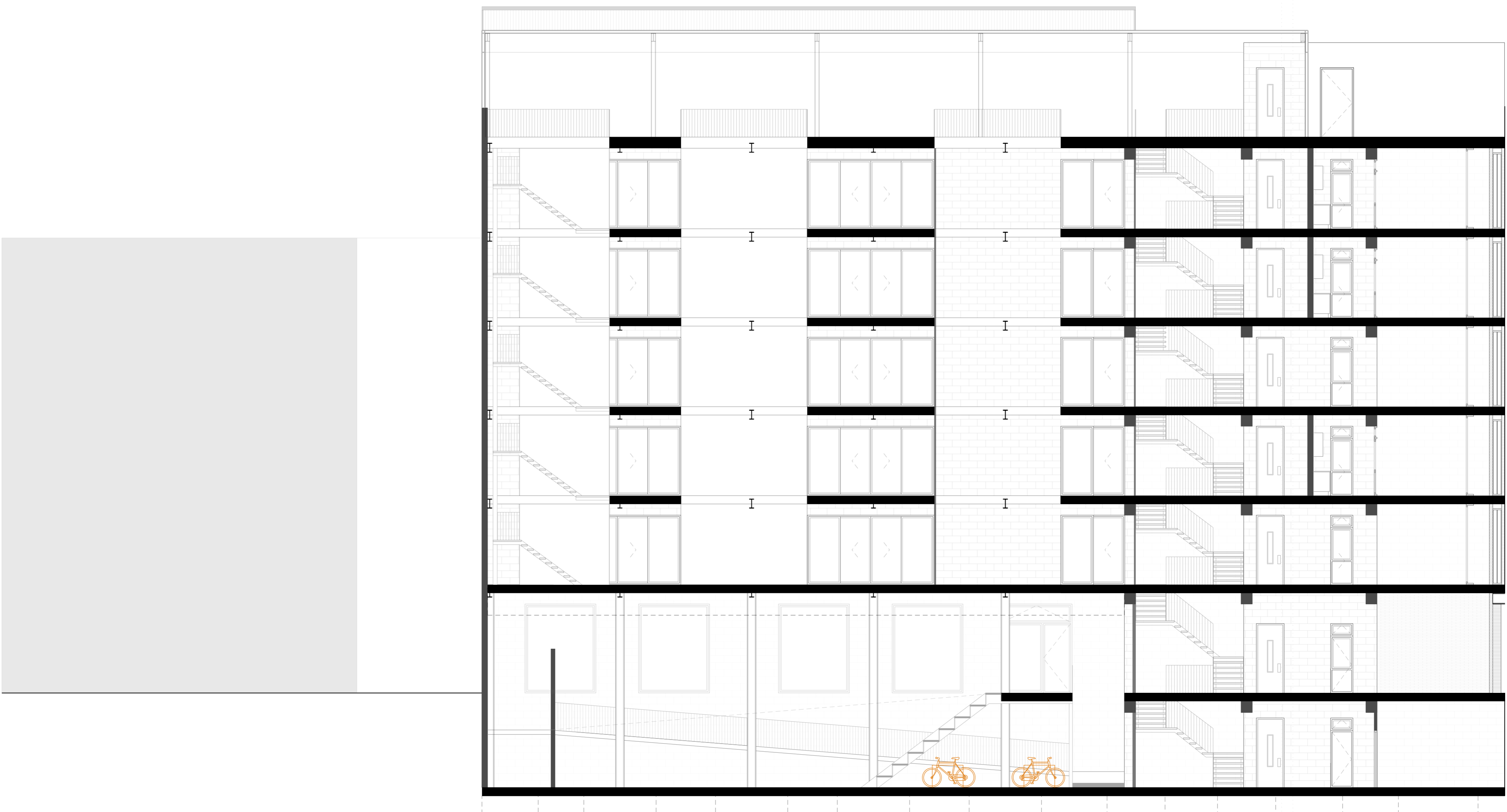
Seccions escala 1:100
