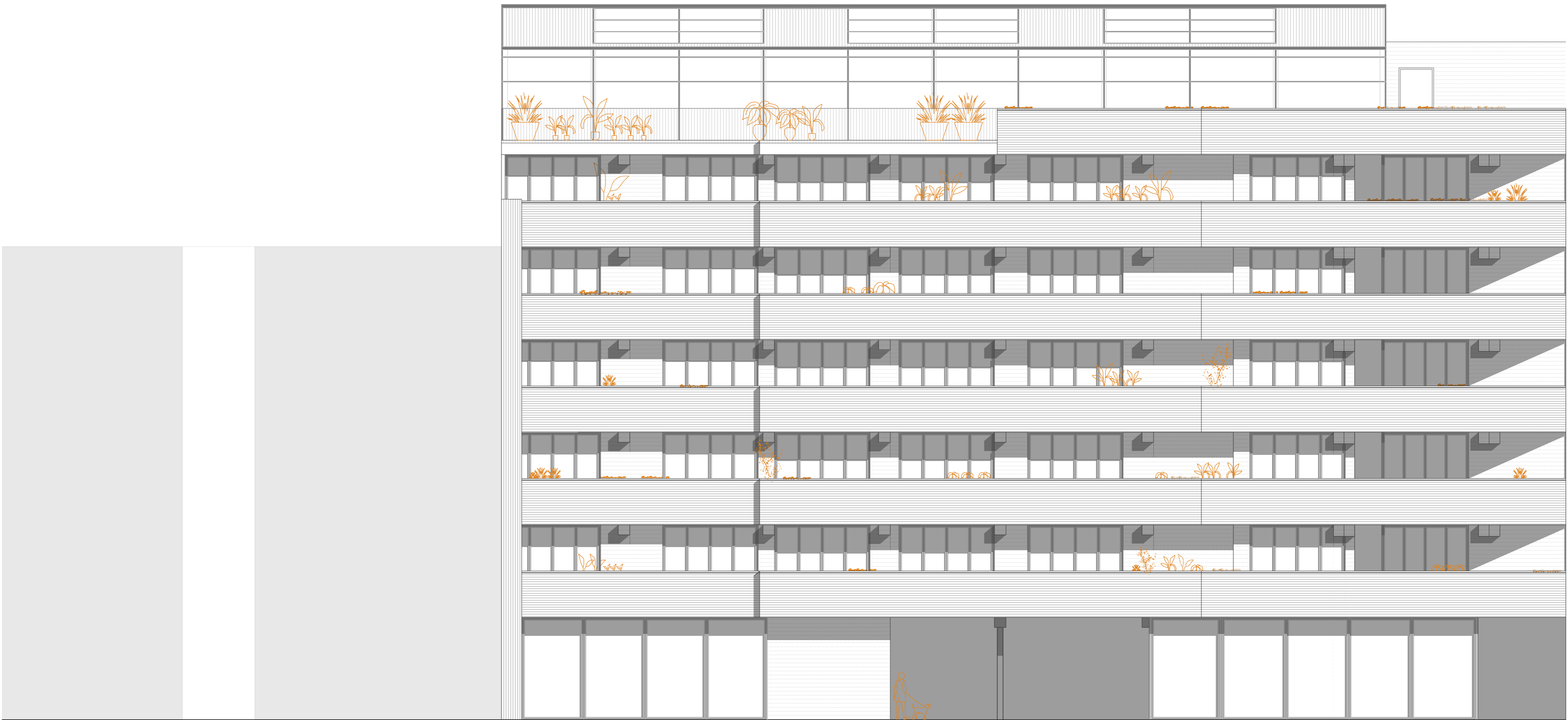
Alçats escala 1:100
