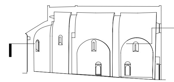
ESGLÉSIA DE SANT PERE DE CASSERRES PLANTA A NIVELL DE LES FINESTRES
