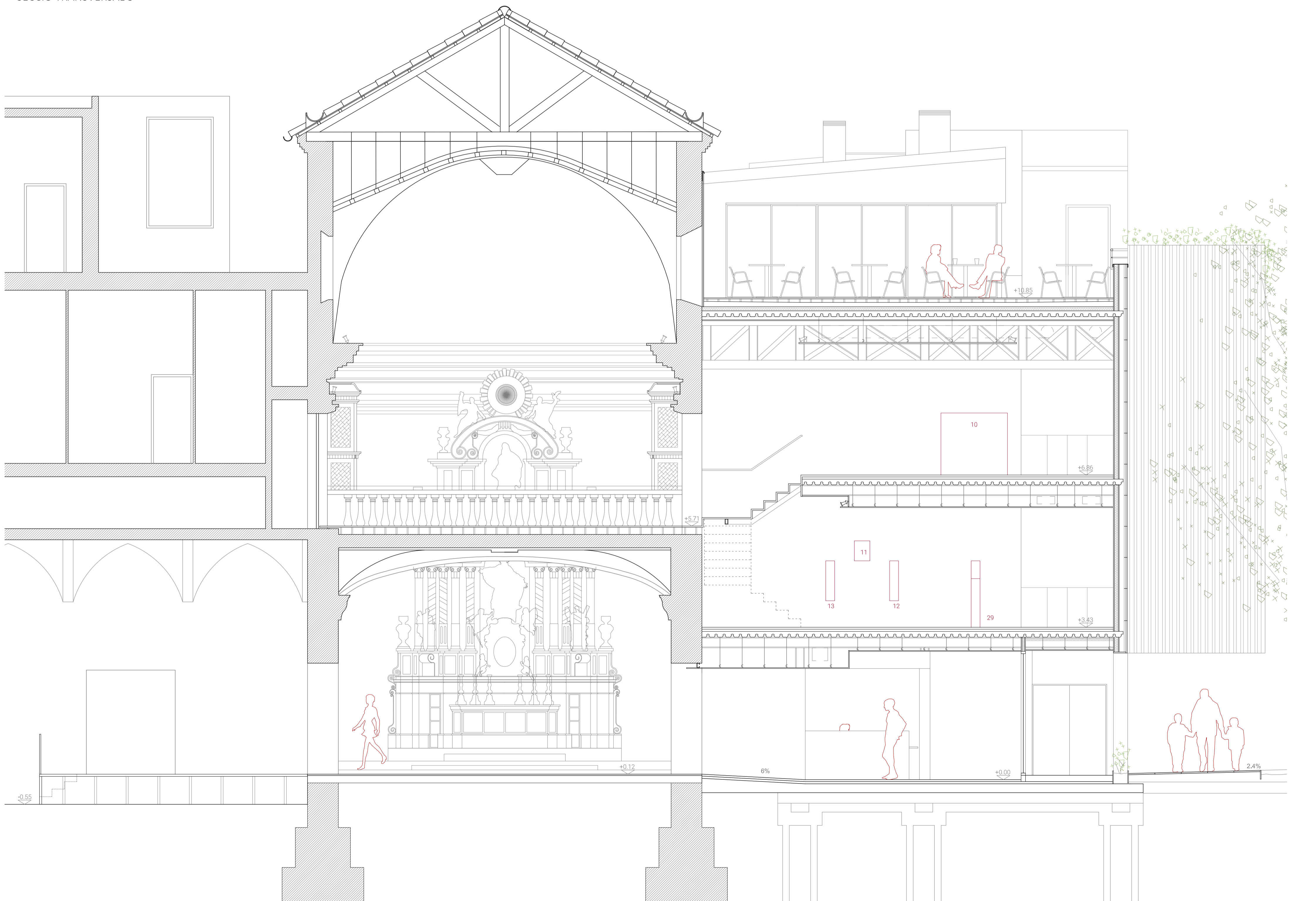
E 1:50
