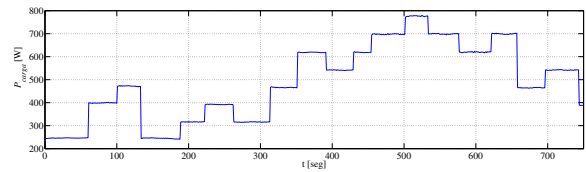
Fig. 5. Potencia demandada por la carga
