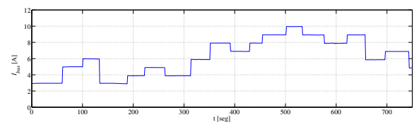
Fig. 7. Corriente en la carga
