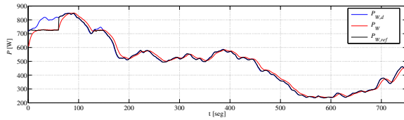
Fig. 8. Potencia disponible y entregada al bus de continua
