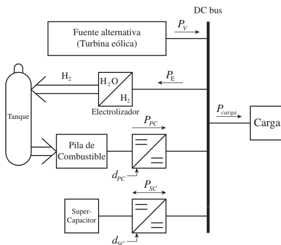
Fig. 1. Diagrama en bloques del sistema híbrido
