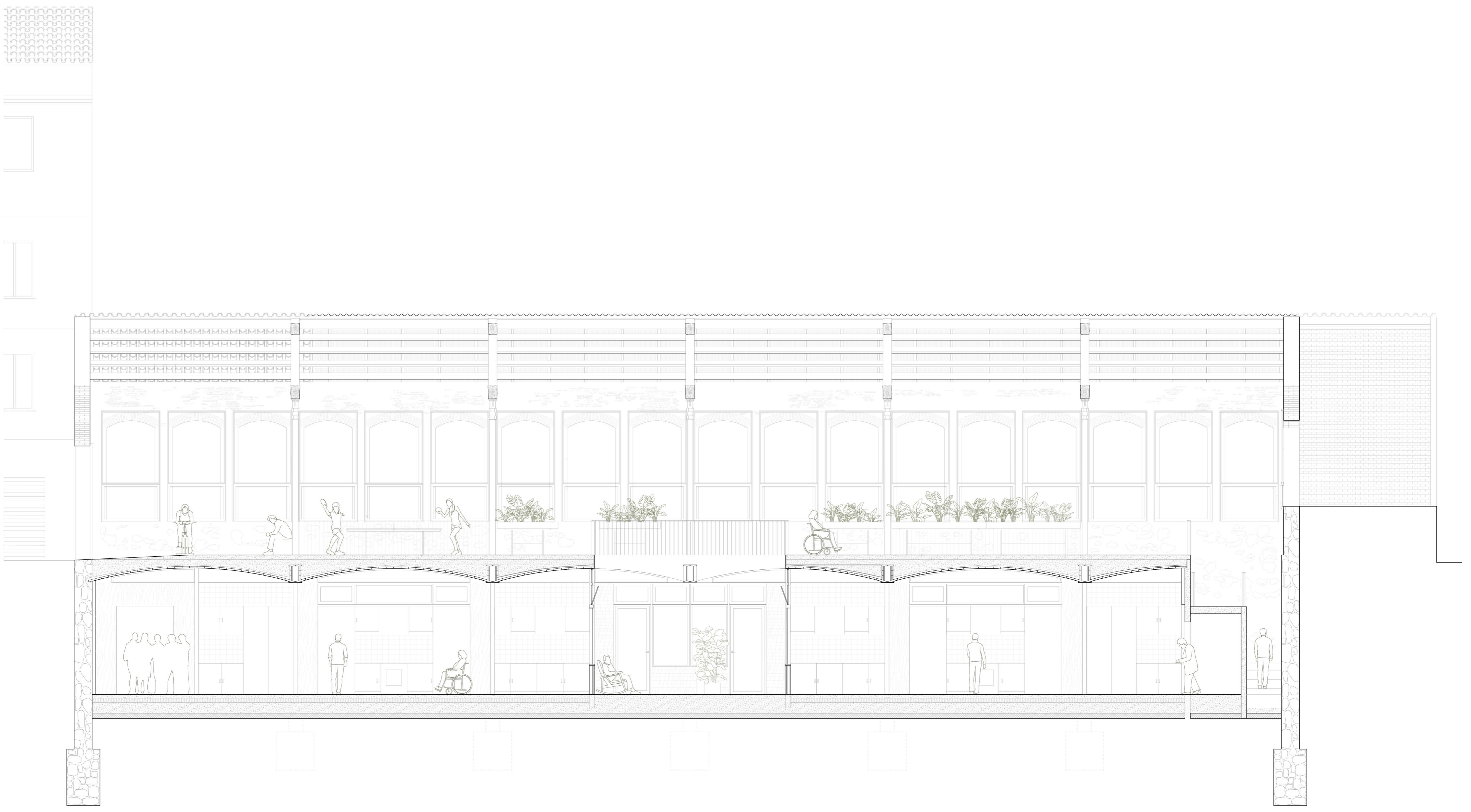
Secció Longitudinal K - K'
