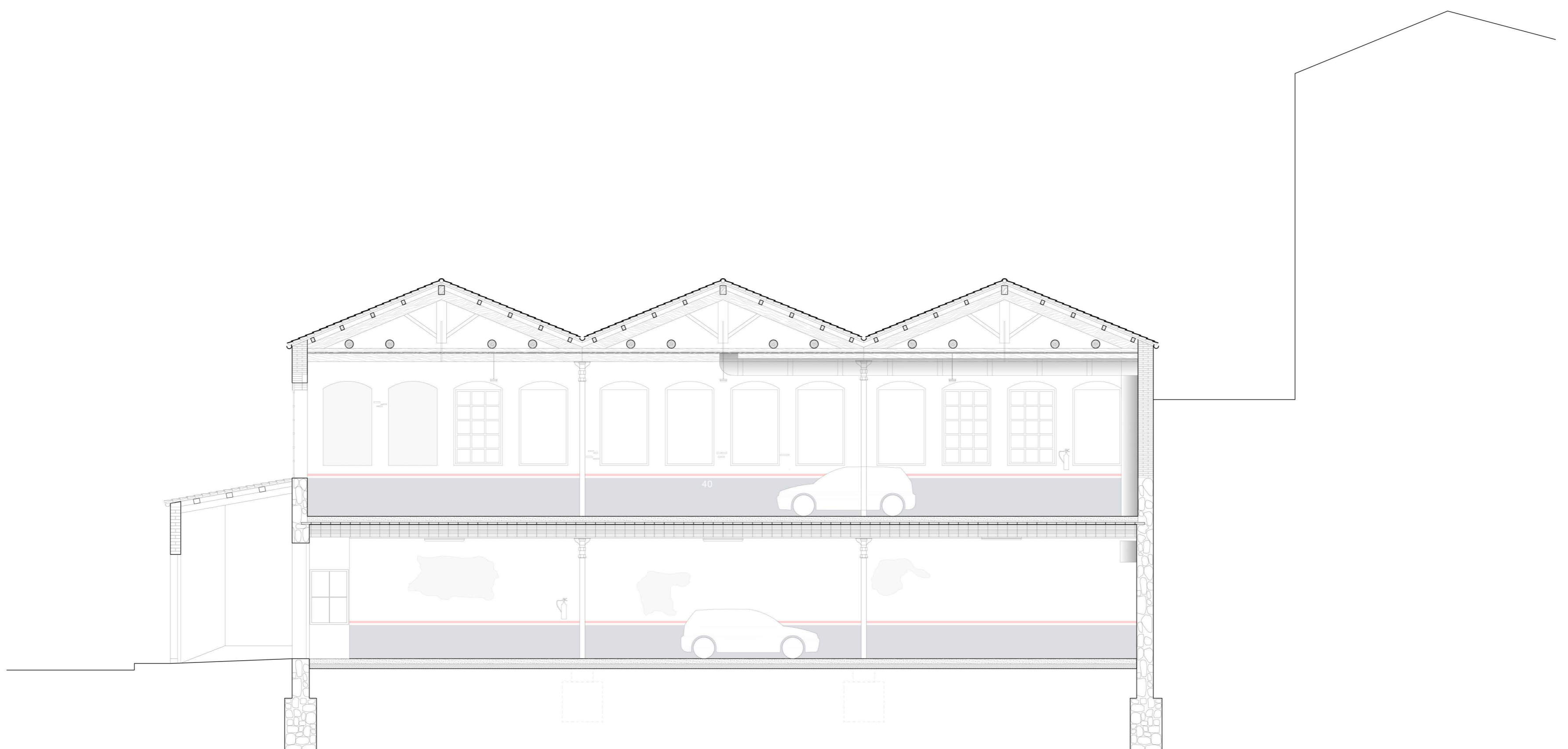
Secció Transversal B - B'
