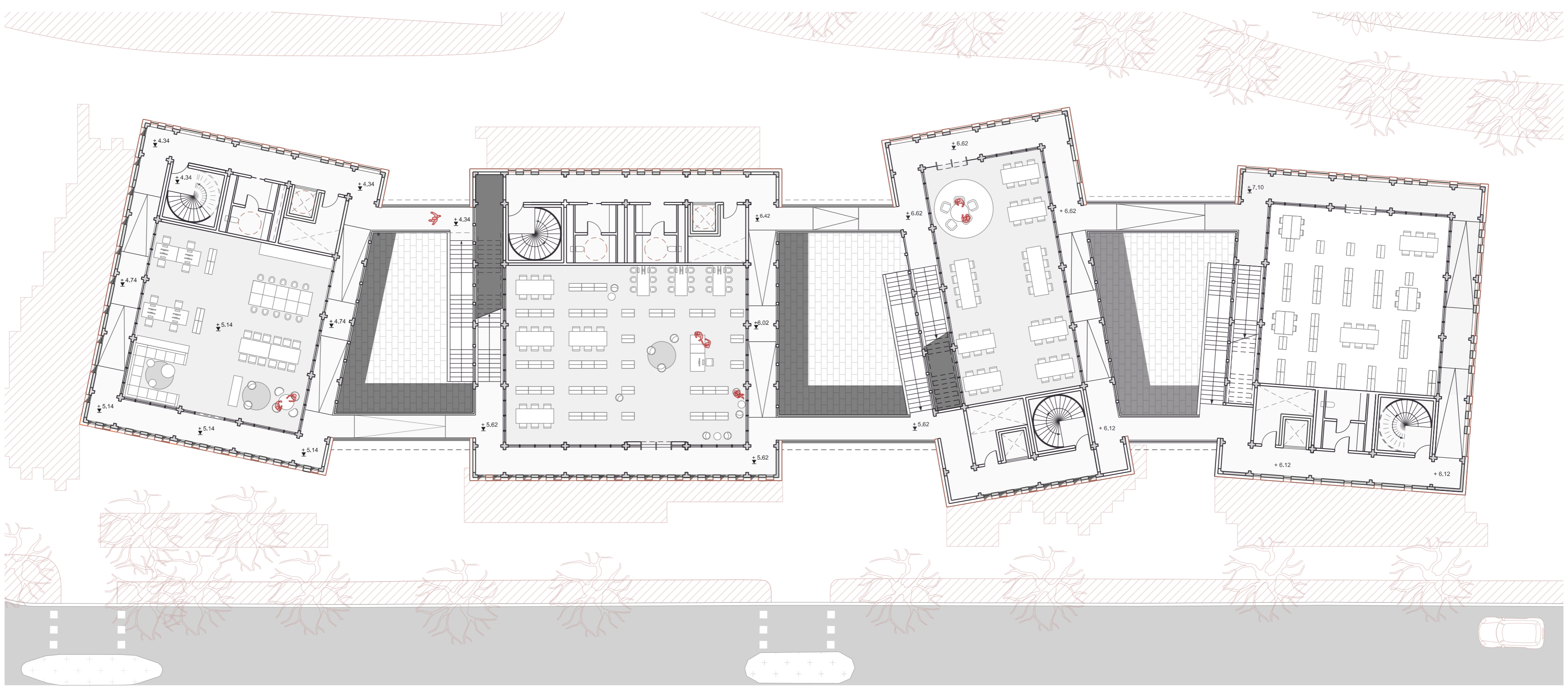
Planta primera 0 2 4 8 10
