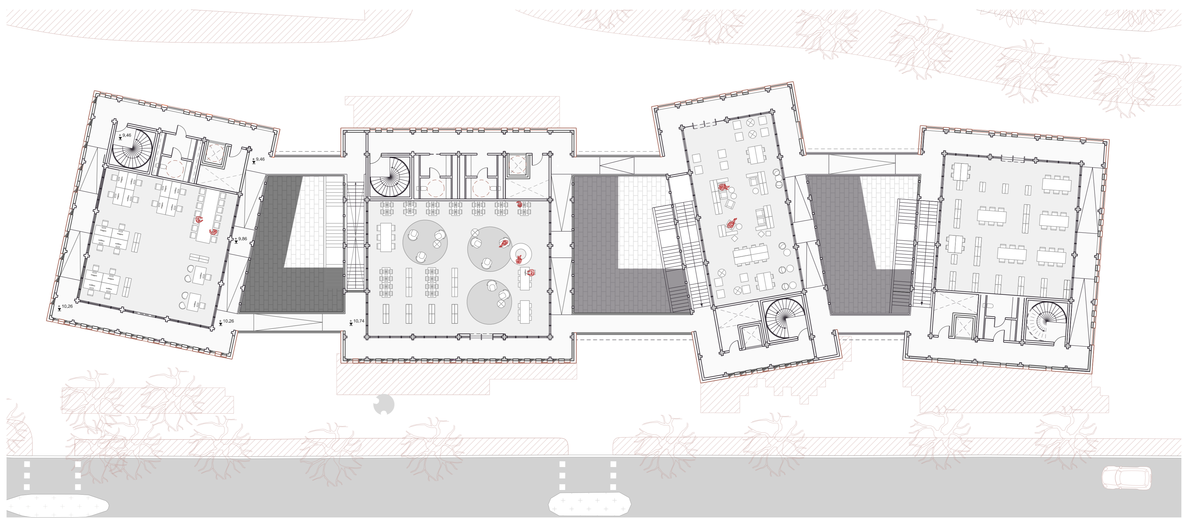
Planta segona 0 2 4 8 10
