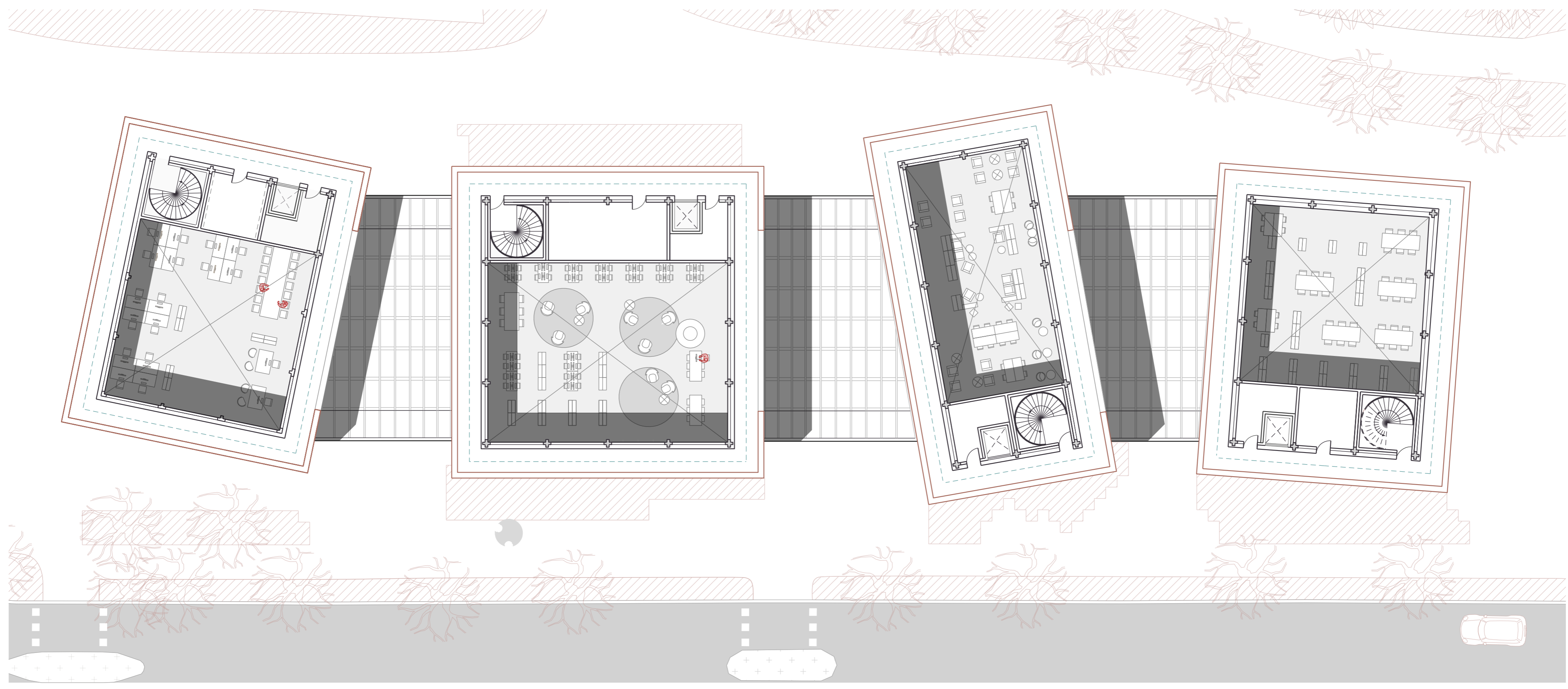
Planta tercera - Sota coberta 0 2 4 8 10
