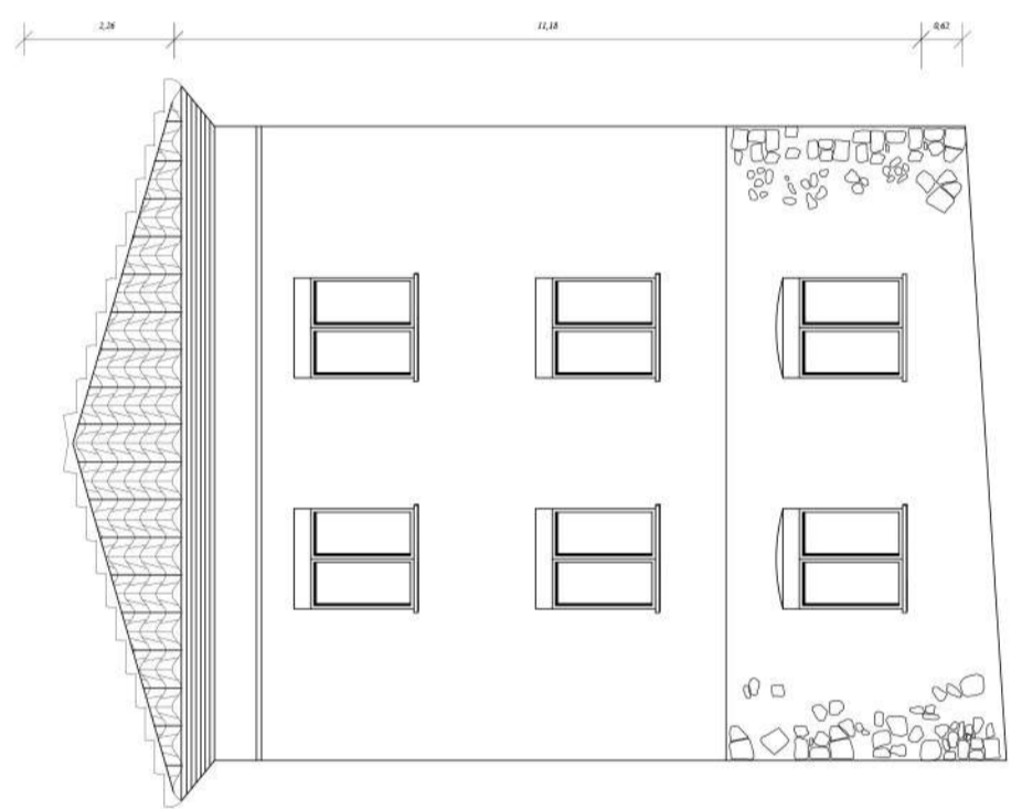
Fachada 2 - Norte -
