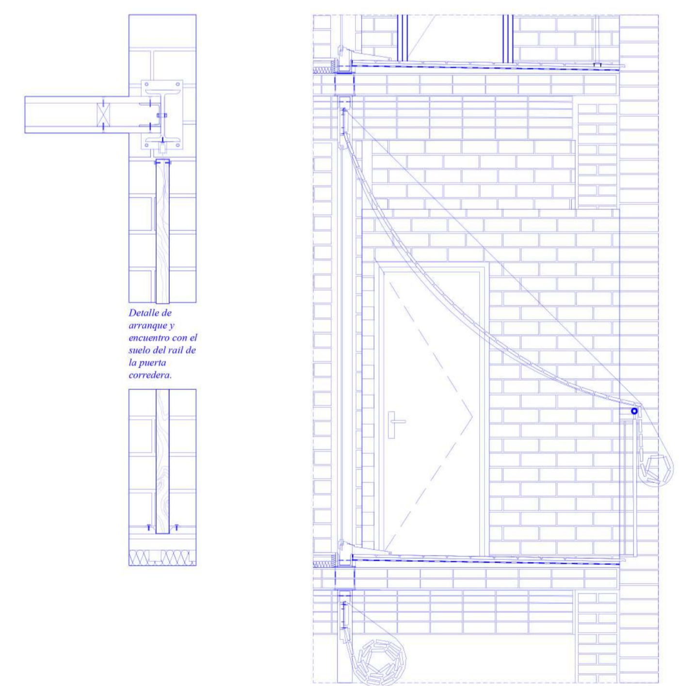
Sección por la galería.
