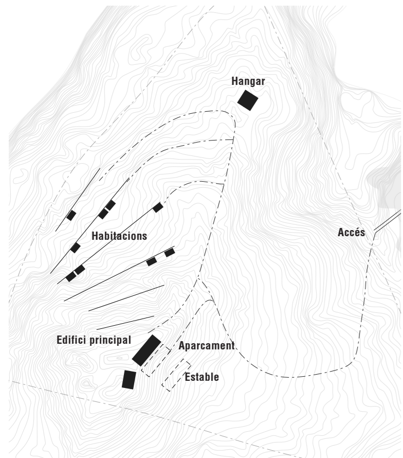
Figura 6.2 Esquema del programa
